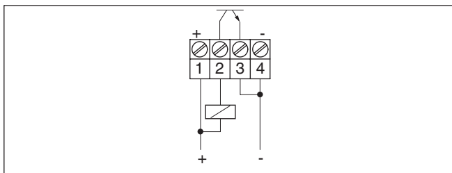
Fig. 11: Comportement NPN
