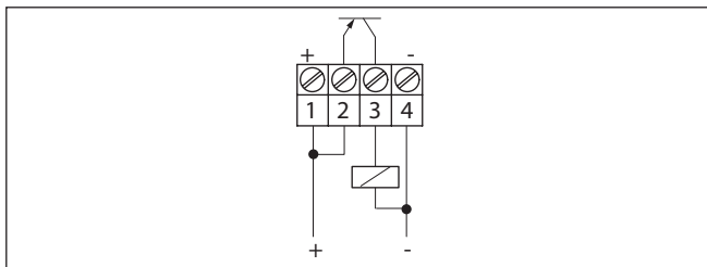
Fig. 12: Comportement PNP
