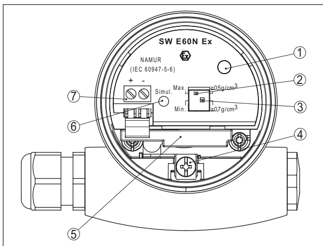
Fig. 10: Compartiment électronique et de raccordement de boîtier à chambre unique
