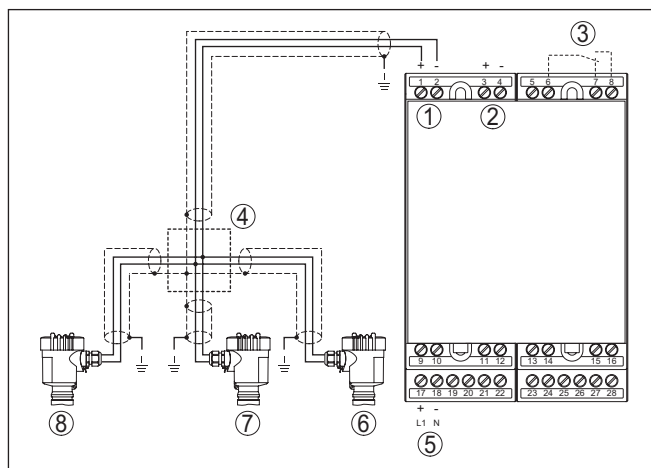
Fig. 3: Aansluitvoorbeeld VEGASCAN 693 met 2-draads sensoren
