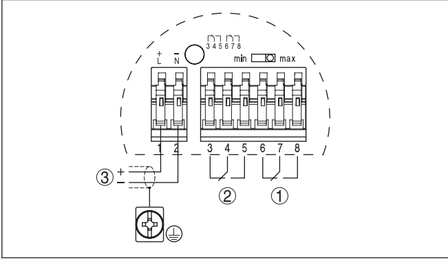
插图. 9: 接线图
