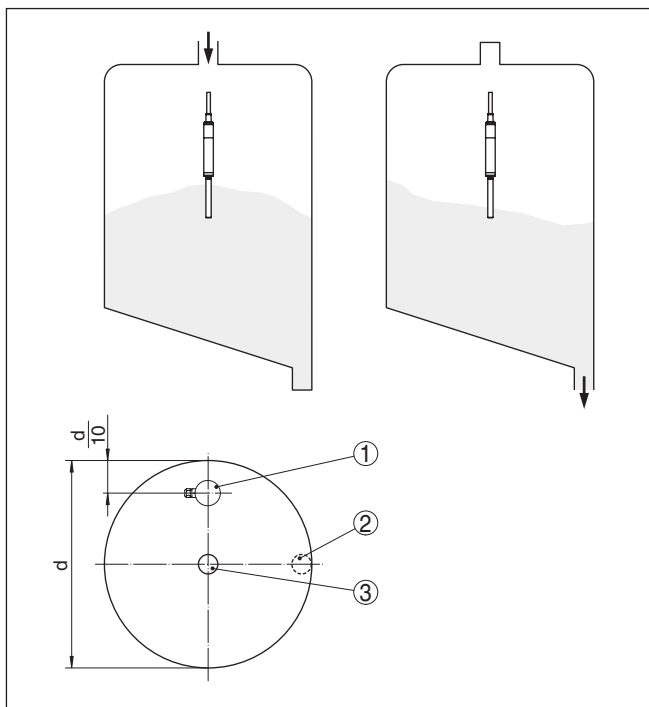
Fig. 4: Vullen in het midden, afvoer aan de zijkant
