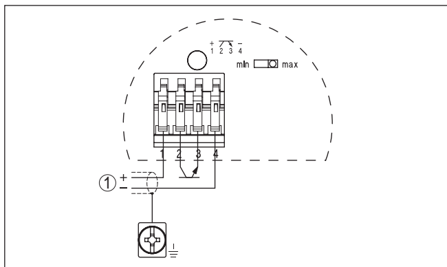
Fig. 9: Wiring plan
