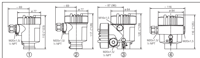
Figura 33: Esecuzioni della custodia
