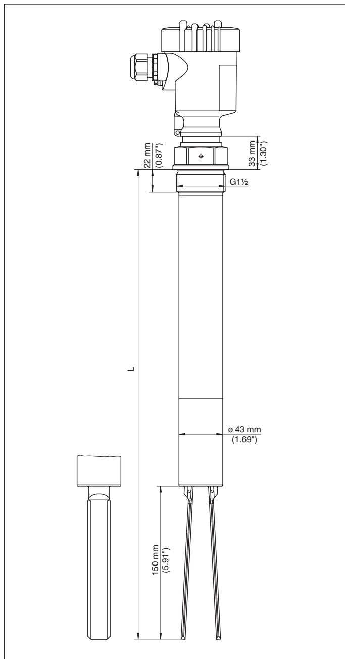
Figura 42: VEGAWAVE 63 - Esecuzione filettata G1 1/2
