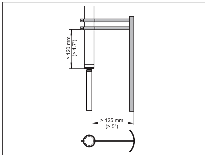
Figura 21: Lamiera di protezione contro danneggiamenti
