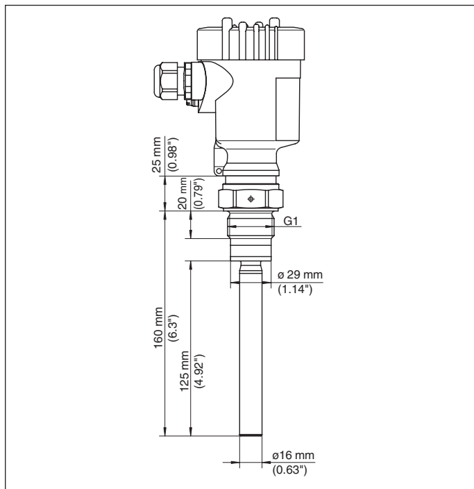
Figura 34: VEGA 61 - Esecuzione filettata G1
