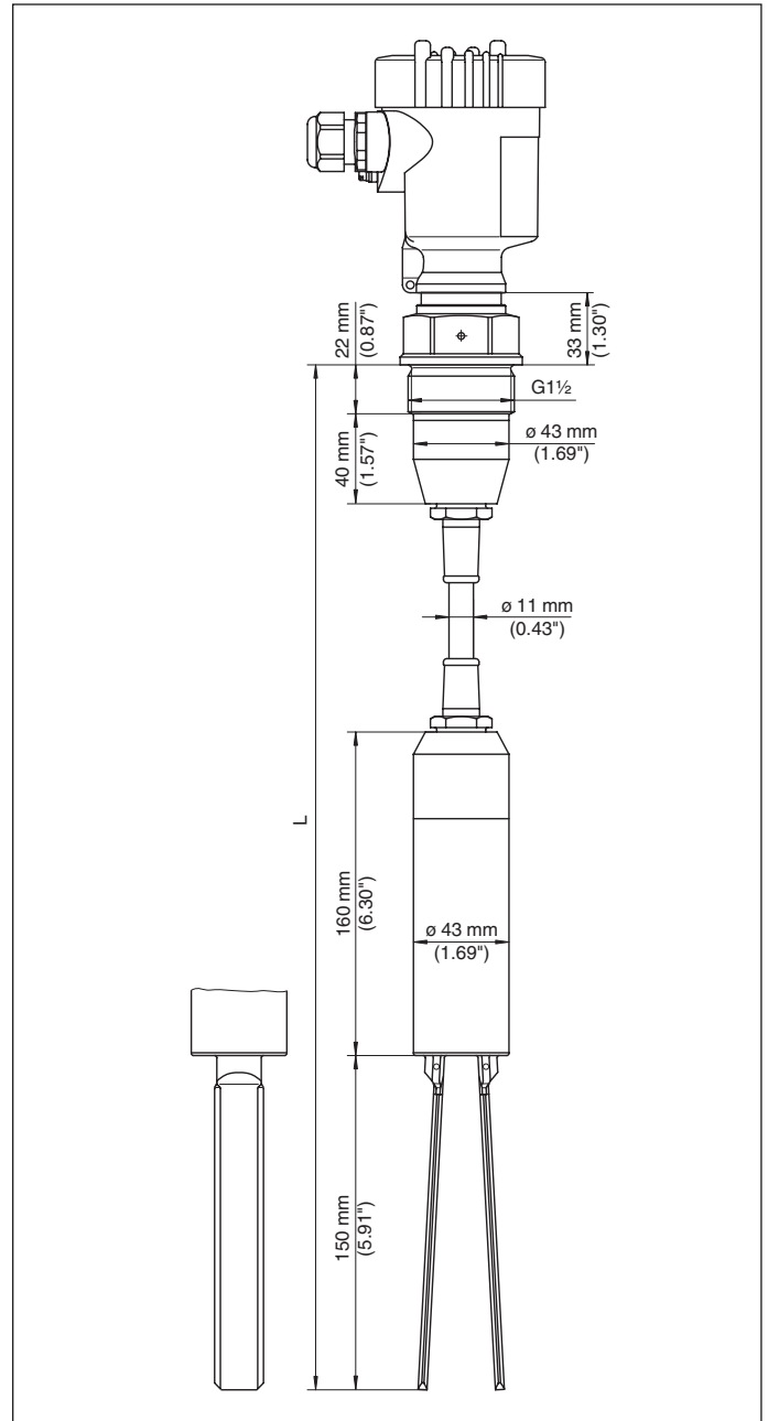
Figura 41: VEGAWAVE 62 - Esecuzione filettata G1 1/2
