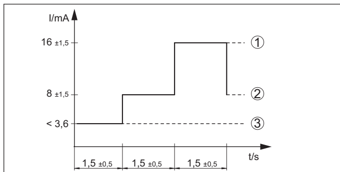
Figura 32: Diagramma di svolgimento del test di funzionamento - Elettronica bifilare
