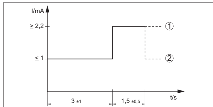
Figura 31: Diagramma di svolgimento del test di funzionamento - Elettronica NAMUR
