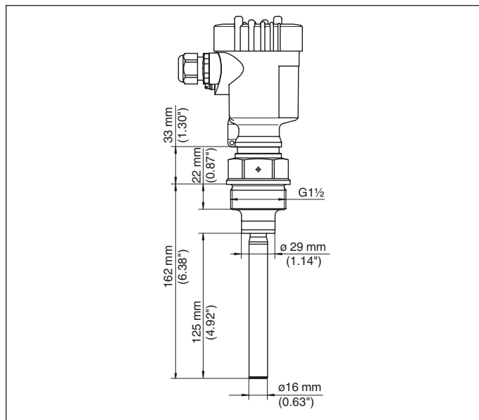
Figura 35: VEGA 61 - Esecuzione filettata G1½
