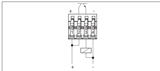
Figura 26: Comportamento PNP
