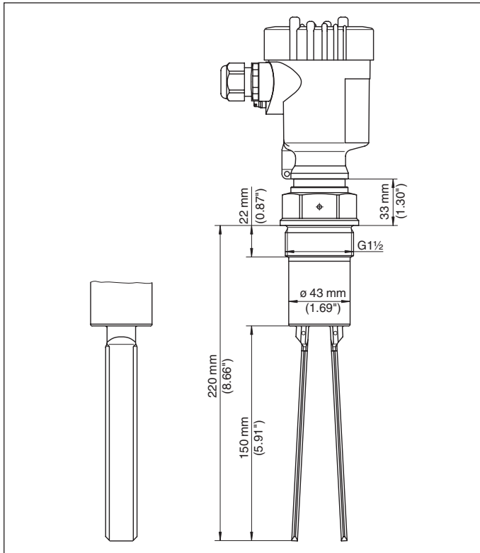
Figura 40: VEGAWAVE 61 - Esecuzione filettata G1 1/2
