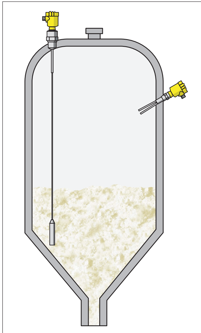
Figura 1: Rilevamento di livello in un silo di stoccaggio di granulati plastici
