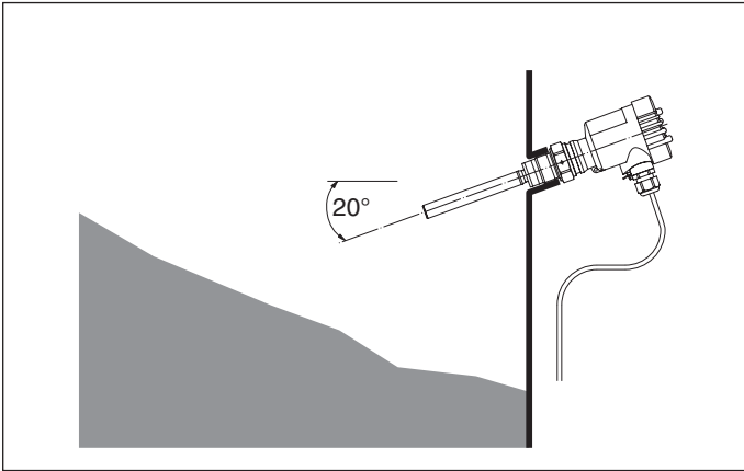
Figura 16: Montaggio orizzontale
