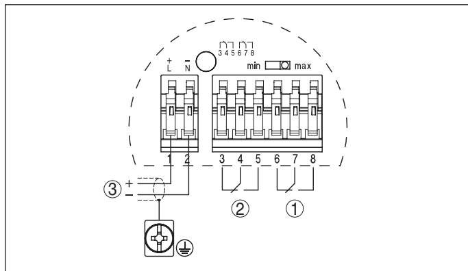
Figura 23: Schema elettrico custodia a una camera
