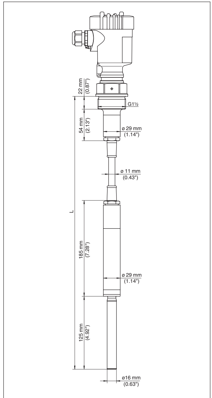
Figura 37: VEGAVIB 62 - Esecuzione filettata G1 1/2
