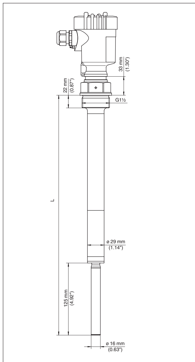
Figura 39: VEGAVIB 63 - Esecuzione filettata G1½
