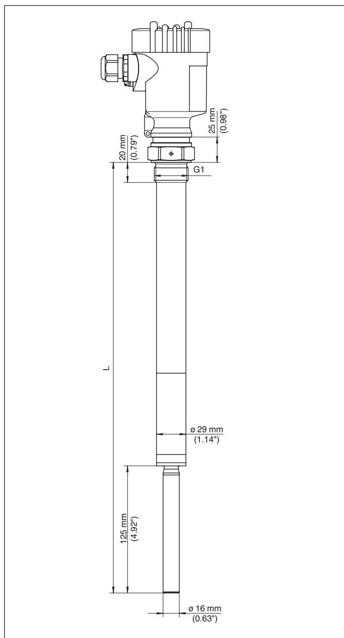
Figura 38: VEGAVIB 63 - Esecuzione filettata G1
