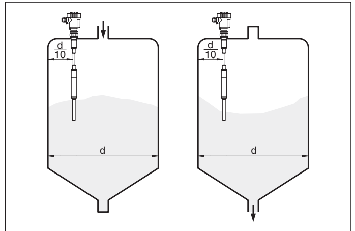
Figura 18: Carico e scarico centrali
