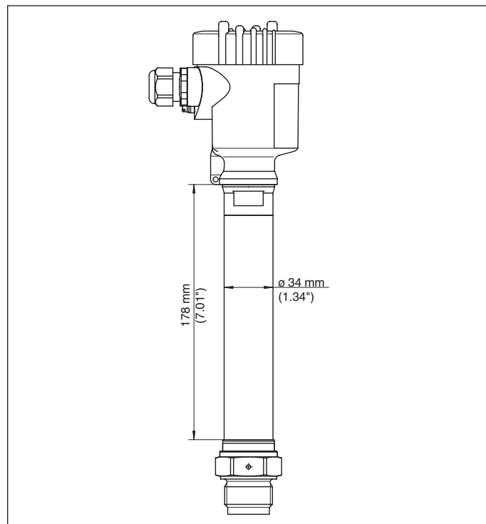
Figura 43: Dissipatore termico (solo per VEGAVIB 61, 63 e VEGAWAVE 61, 63)
