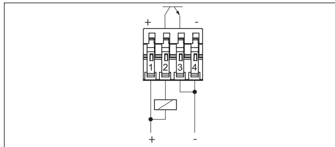
Figura 25: Comportamento NPN
