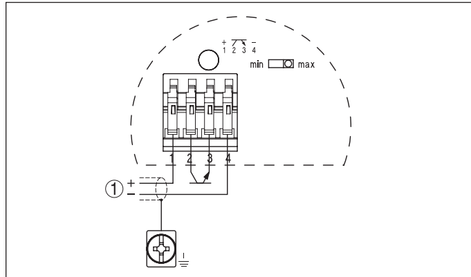
Figura 24: Schema elettrico custodia a una camera
