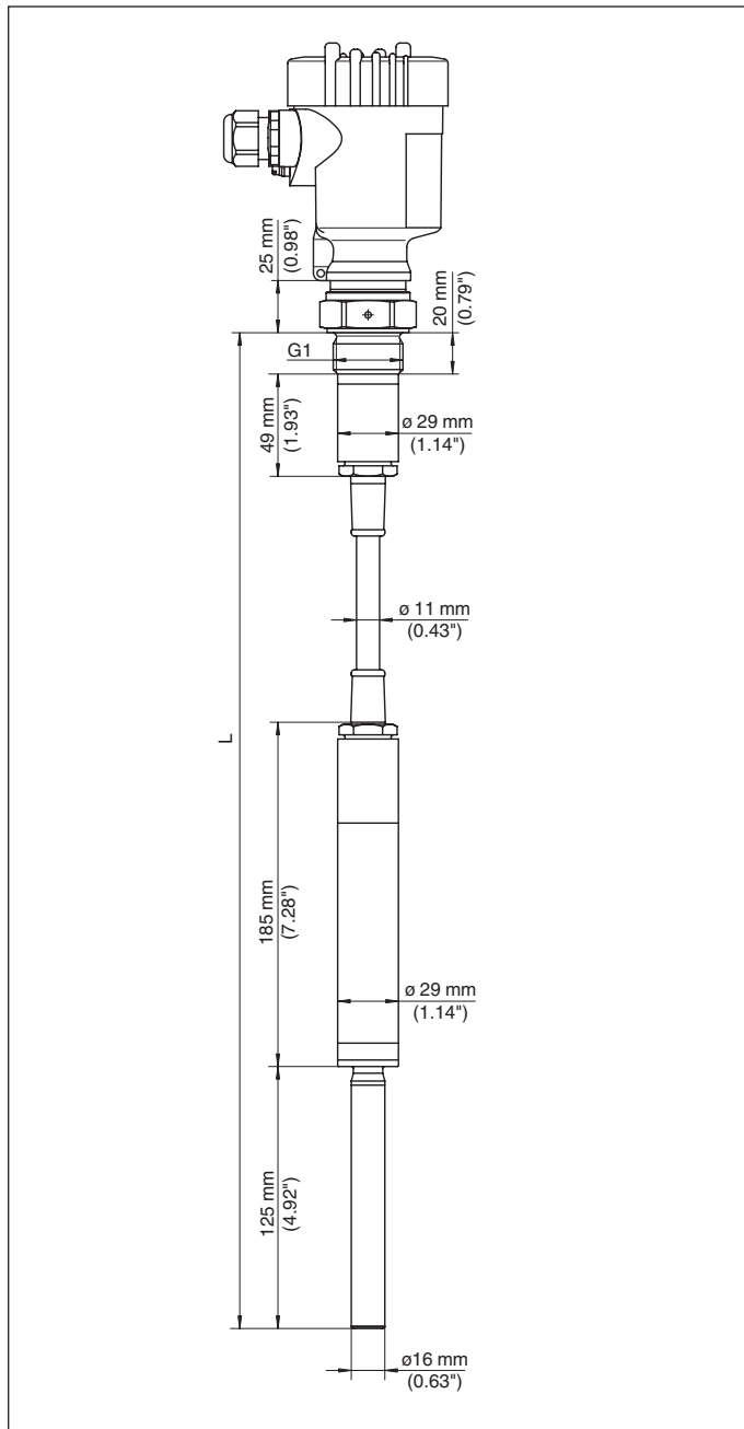
Figura 36: VEGAVIB 62 - Esecuzione filettata G1
