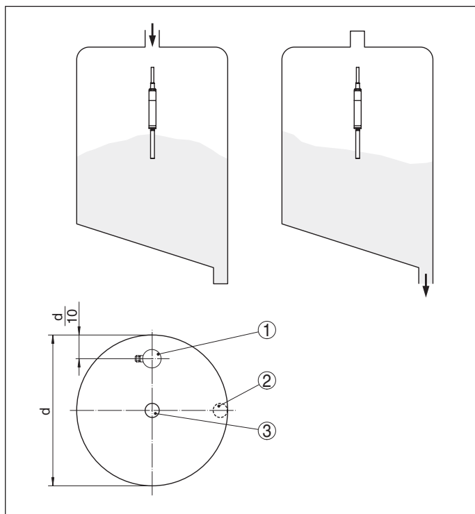
Figura 19: Carico centrale, scarico laterale
