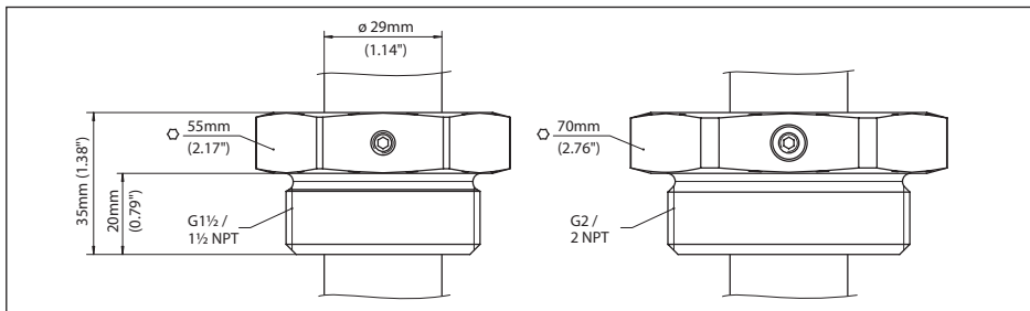
Fig. 2: Borgkoppeling ARV-VB63.1 drukloos voor VEGA VIB 63
