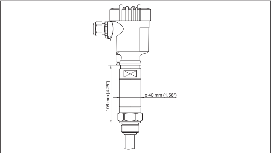
Res. 21: Sıcaklık adaptörü
