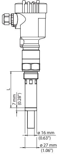
Res. 22: VEGACAP 62, ör. şiddetli yoğunlaşma karşış yalıtımlı boru
