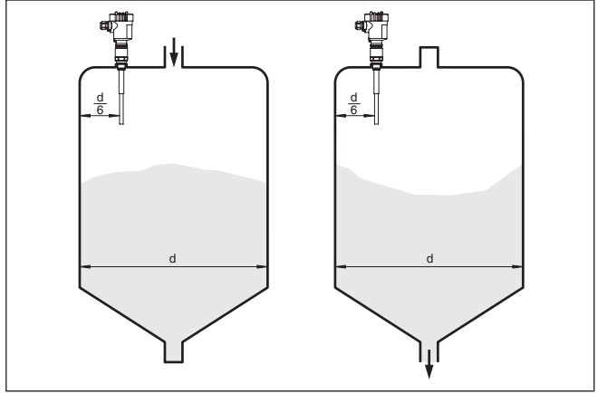
Res. 7: Doldurma ve boşaltma ortaya
