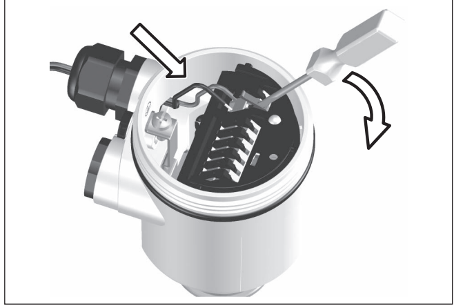
Res. 9: Bağlantı prosedürü 5 ve 6
