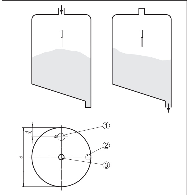
Res. 8: Doldurma ortaya, boşaltma yana
