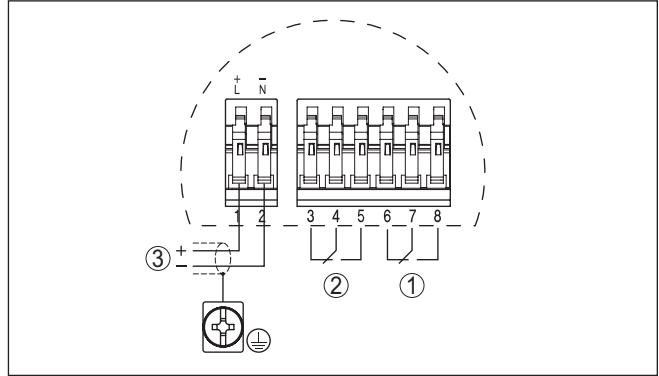
Res. 12: Bağlantı şeması
