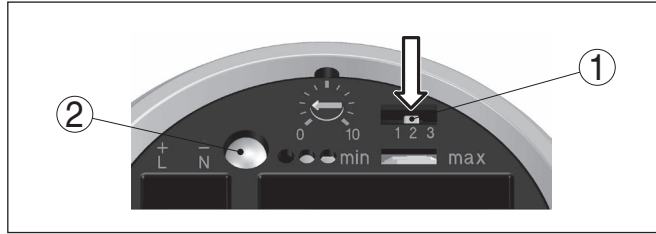
Res. 16: Kompanzasyon düğmesi
