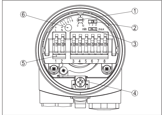
Res. 13: Röle çıkışlı elektronik modül
