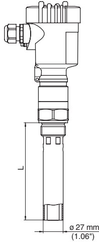
Res. 23: VEGACAP 62, dielektrite değeri küçük olduğunda veya lineerizasyon için
