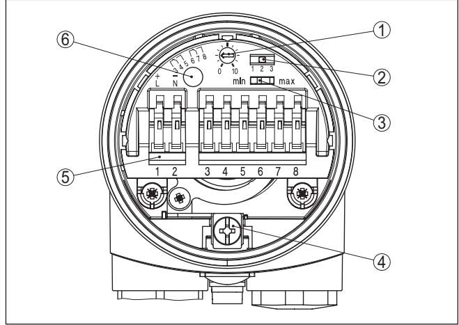
Res. 11: Elektronik bölme ve bağlantı bölgesi
