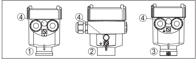
Res. 10: Tek bölmeli gövde malzeme çeşitleri
