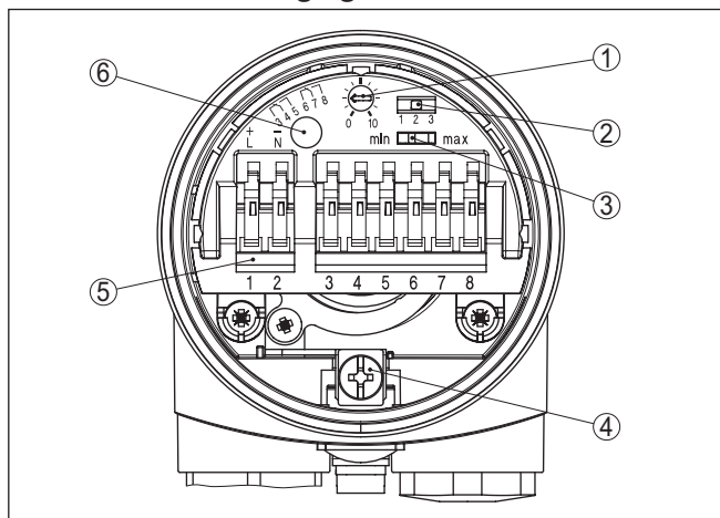
Fig. 11: Électronique avec sortie relais
