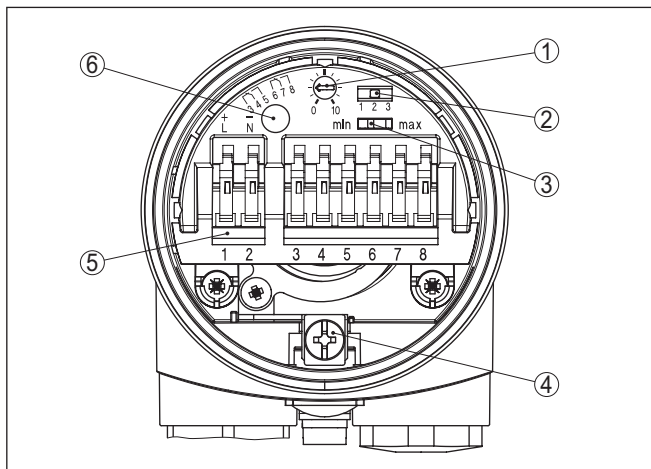
Fig. 9: Compartiment électronique et de raccordement
