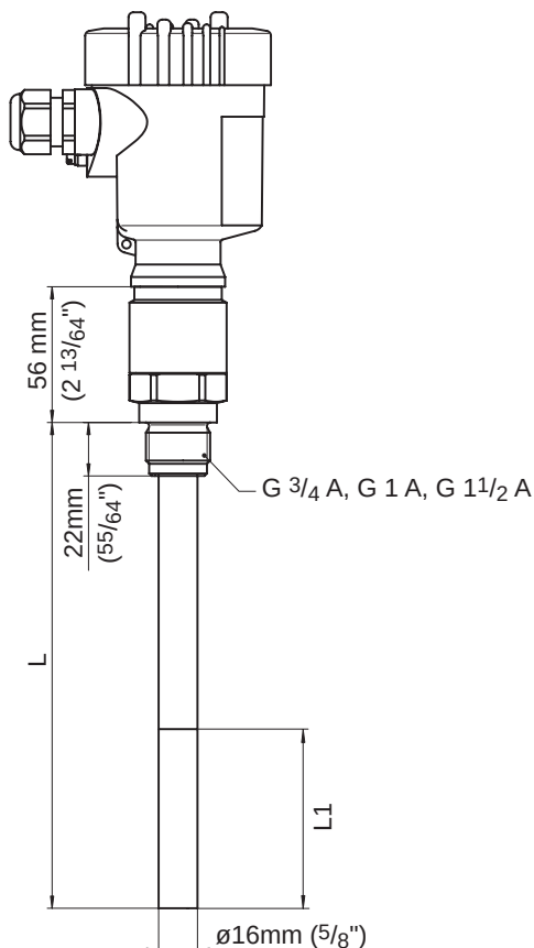
Abb. 17: VEGACAP 64, Gewindeausführung G1 (ISO 228 T1)
