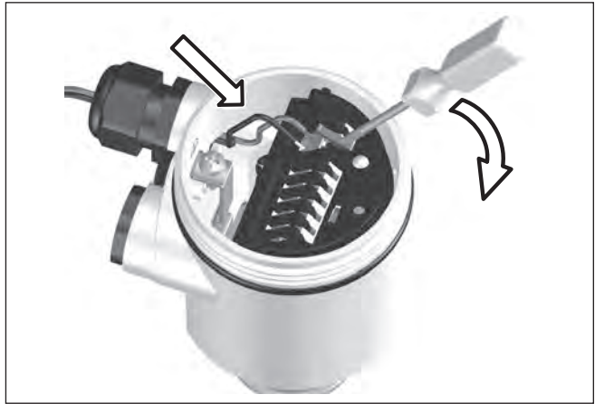
Abb. 7: Anschlusschritte 5 und 6
