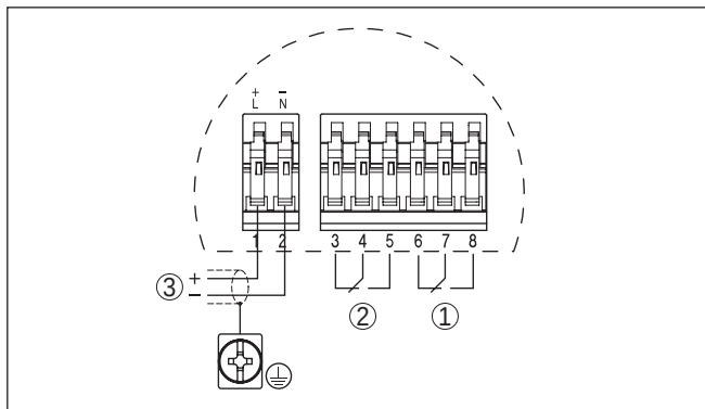
Abb. 10: Anschlussplan
