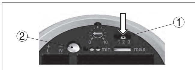
Abb. 14: Kompensationstaster
