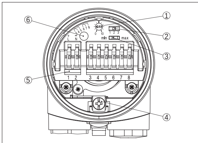
Abb. 9: Elektronik- und Anschlussraum
