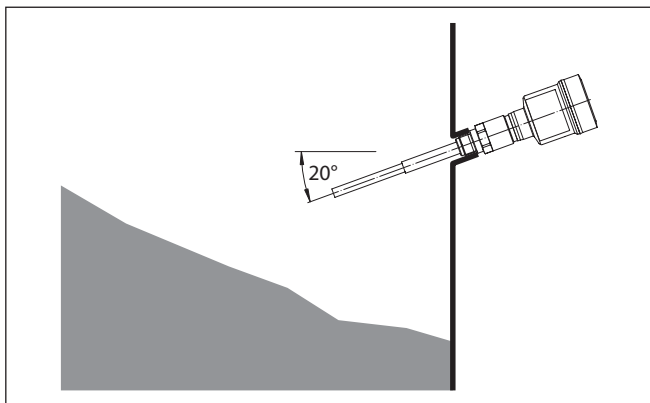
Abb. 6: Waagerechte Montage
