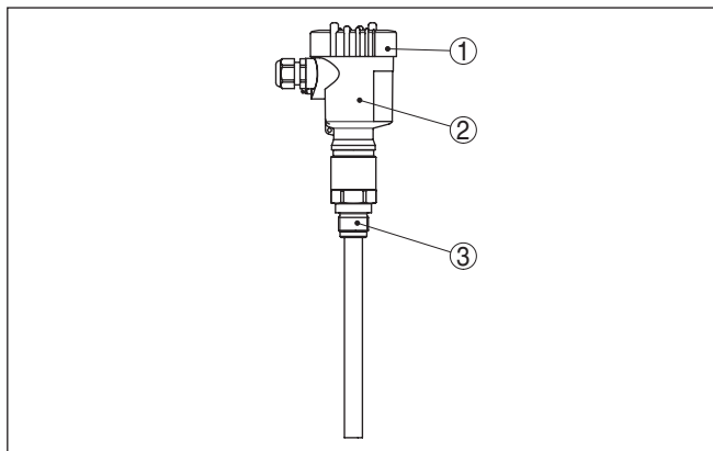
Abb. 1: VEGACAP 64, Stabausführung mit Kunststoffgehäuse
