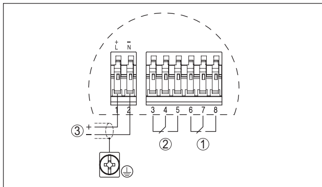
Fig. 10: Aansluitschema
