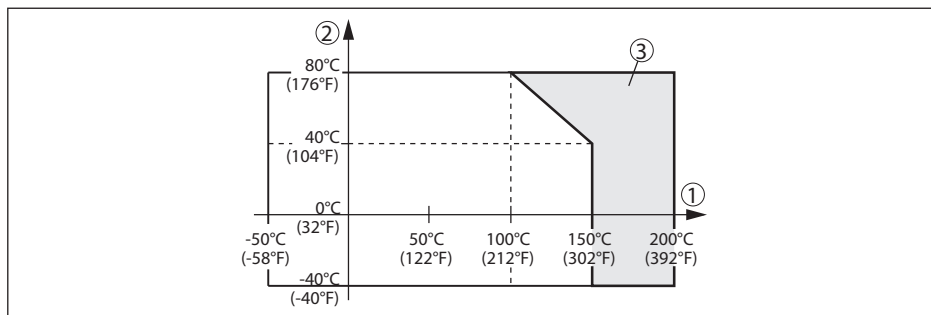
Fig. 15: Omgevingstemperatuur - procestemperatuur
