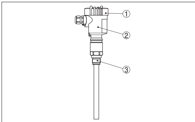
Fig. 1: VEGACAP 64, staafversie met kunststof behuizing
