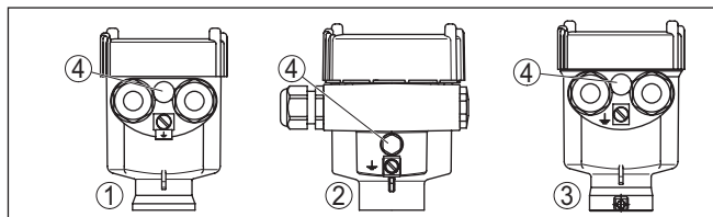
Fig. 8: Materiaalvarianten eenkamerbehuizing
