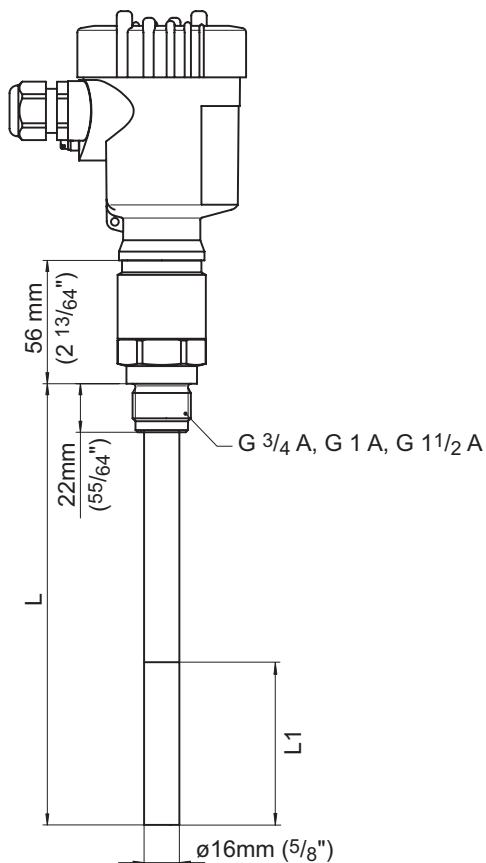
Fig. 17: VEGACAP 64, schroefdraaduitvoering G1 (ISO 228 T1)
