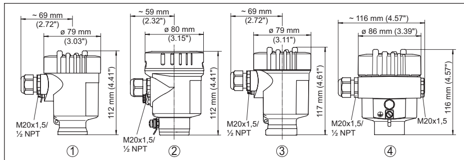
Fig. 16: Uitvoeringen behuizing
