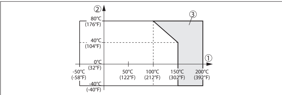
Abb. 15: Umgebungstemperatur - Prozesstemperatur
