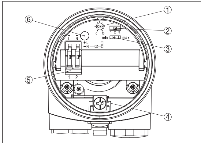
Abb. 11: Elektronikeinsatz - kontaktloser Schalter
