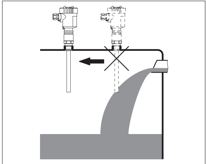
Abb. 5: Einströmendes Medium
