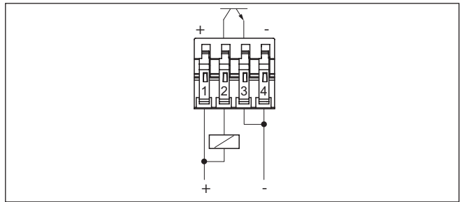
Abb. 11: NPN-Verhalten
