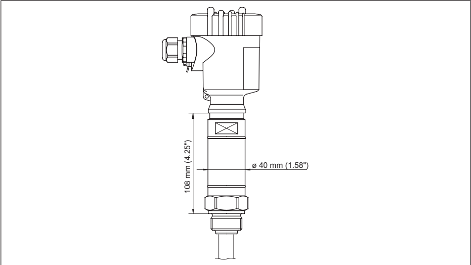
Abb. 22: Temperaturzwischenstück
