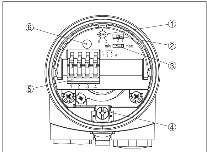
Abb. 14: Elektronikeinsatz - Transistorausgang
