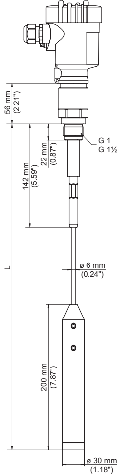
Res. 20: VEGACAP 65, 6 mm (0.236 in) çapında kablolu model, G1 dişli model (ISO 228 T1)
