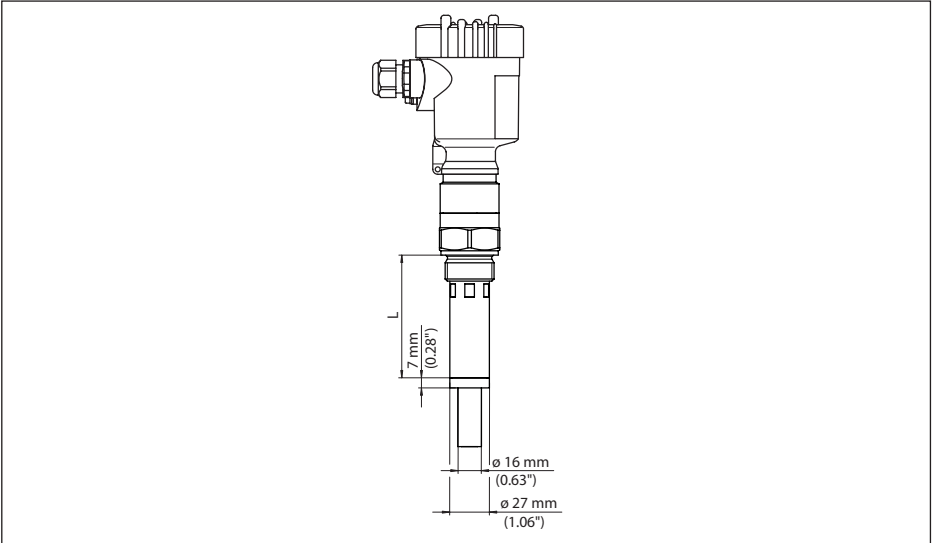
Res. 24: VEGACAP 65, ör. şiddetli yoğunlaşım olmasına karşı yalıtımlı boru
