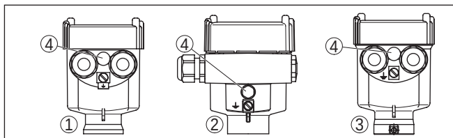
Abb. 9: Werkstoffvarianten Einkammergehäuse
