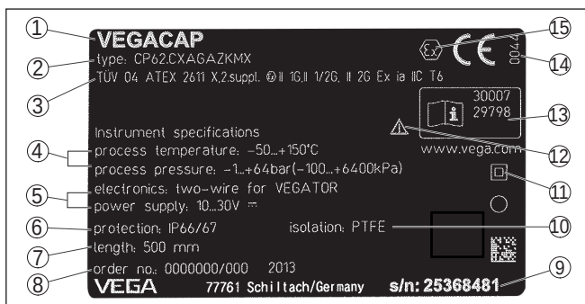
Abb. 2: Aufbau des Typschildes (Beispiel)
