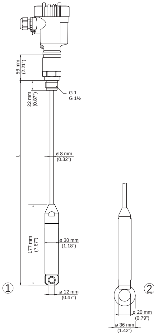
Abb. 18: VEGACAP 66, Gewindeausführung G1 (ISO 228 T1)
