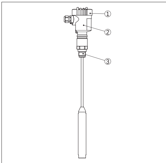
Abb. 1: VEGACAP 66, Seilausführung mit Kunststoffgehäuse
