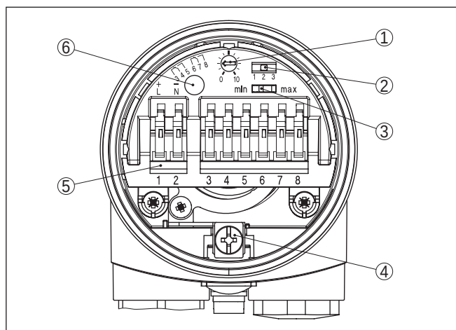
Abb. 12: Elektronikeinsatz - Relaisausgang
