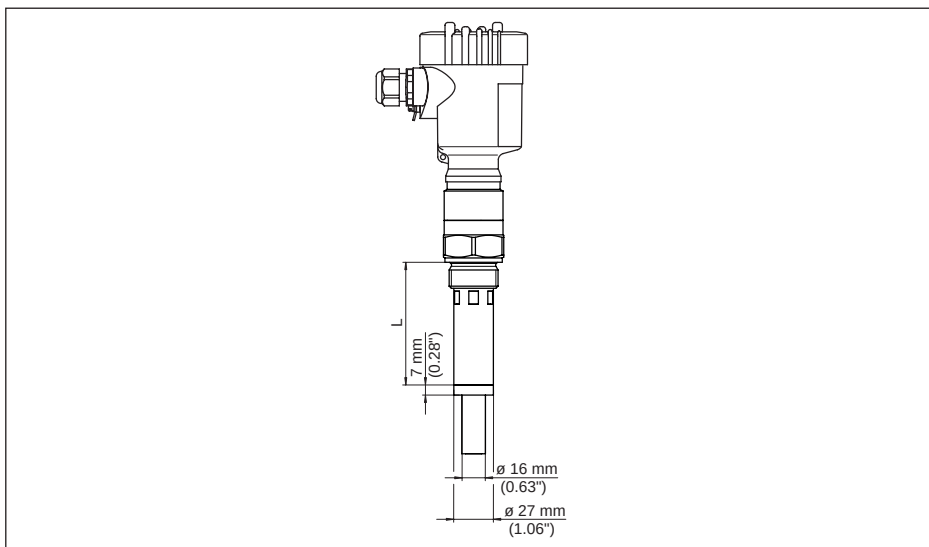
Abb. 19: VEGACAP 66, Abschirmrohr z. B. gegen starke Kondensatbildung
