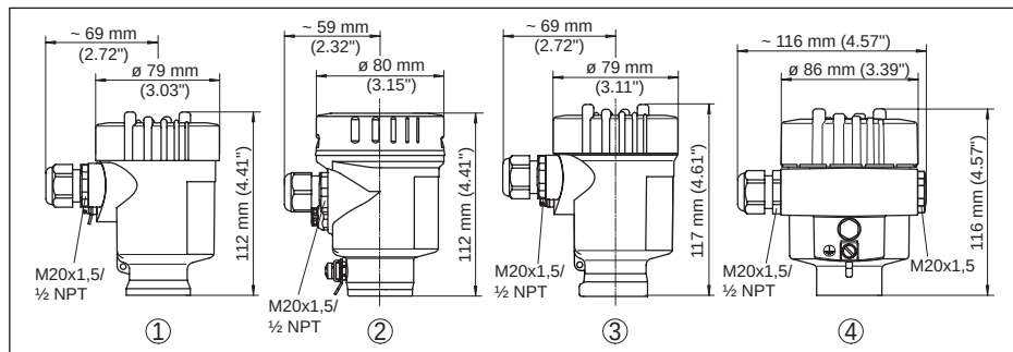
Abb. 17: Gehäuseausführungen
