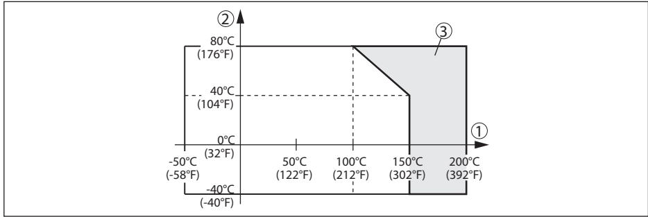
Res. 16: Ortamdaki maddenin sıcaklığı - Proses sıcaklığı
