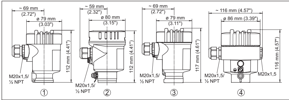
Res. 17: Gövde modelleri
