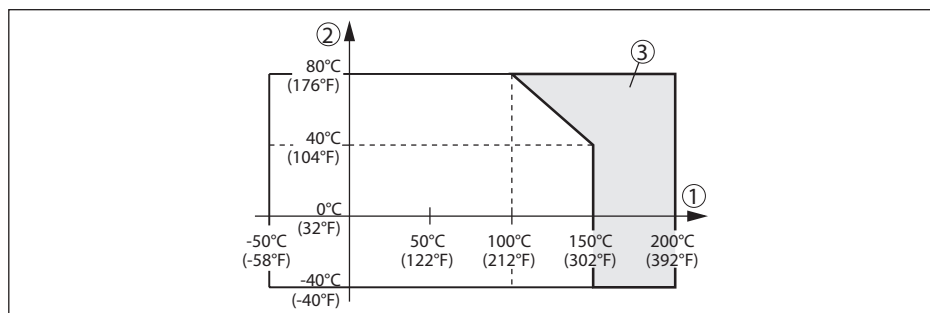
Fig. 16: Omgevingstemperatuur - processtemperatuur
