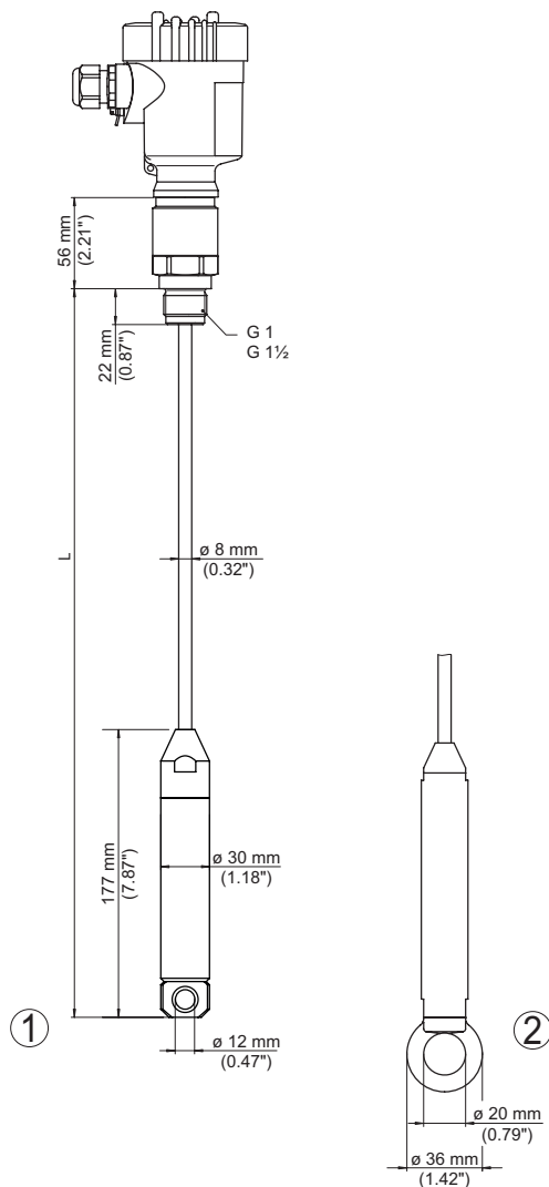
Fig. 18: VEGACAP 66, schroefdraaduitvoering G1 (ISO 228 T1)
