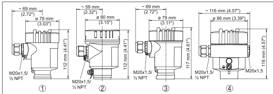
Fig. 17: Uitvoeringen behuizing
