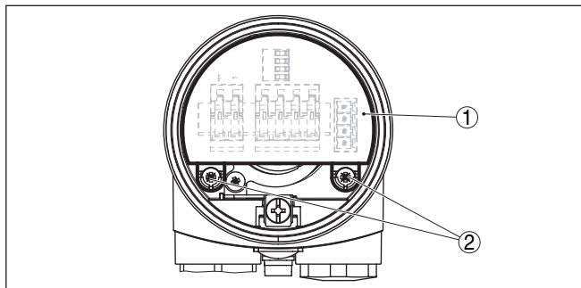
Fig. 14: Bevestigingsschroeven losmaken
