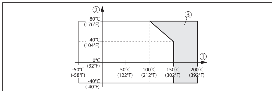
Fig. 30: Omgevingstemperatuur - procestemperatuur
