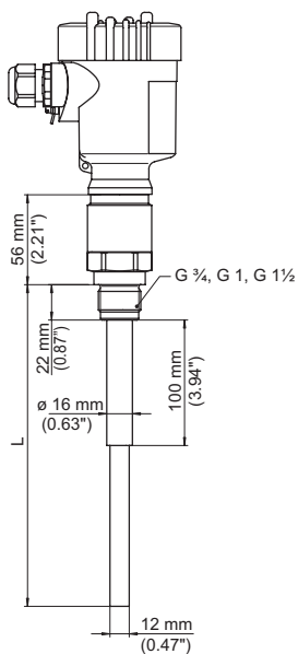
Fig. 34: VEGACAL 62, schroefdraaduitvoering G1 (ISO 228 T1)
