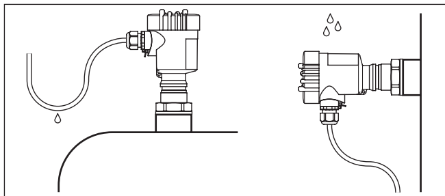
Fig. 5: Maatregelen tegen het binnendringen van vocht
