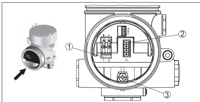
Fig. 14: Aansluitruimte - tweekamerbehuizing
