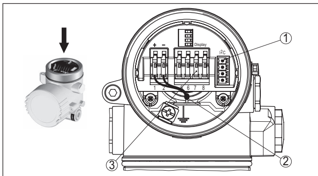
Fig. 17: Elektronicar ruimte - tweekamerbehuizing
