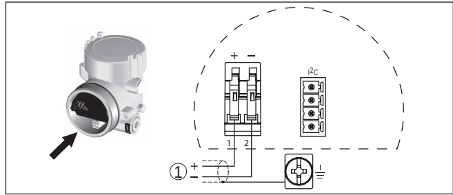
Abb. 15: Anschlussplan - Zweikammergehäuse
