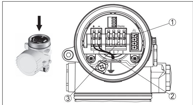
Abb. 17: Elektronikraum - Zweikammergehäuse
