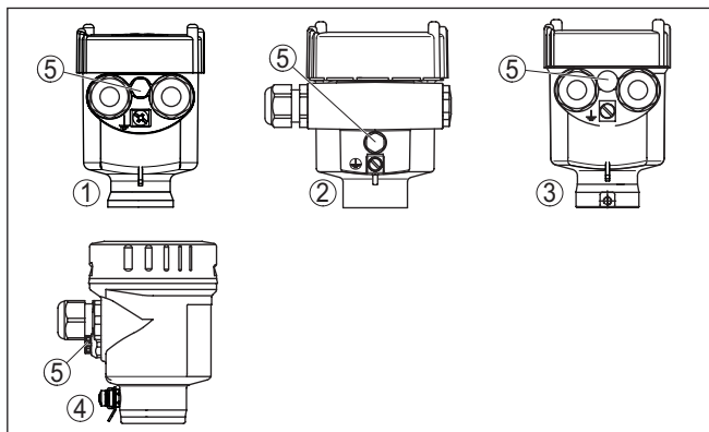
Abb. 9: Werkstoffvarianten Einkammergehäuse
