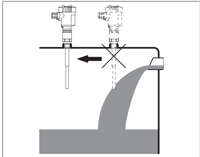
Abb. 7: Einströmendes Medium
