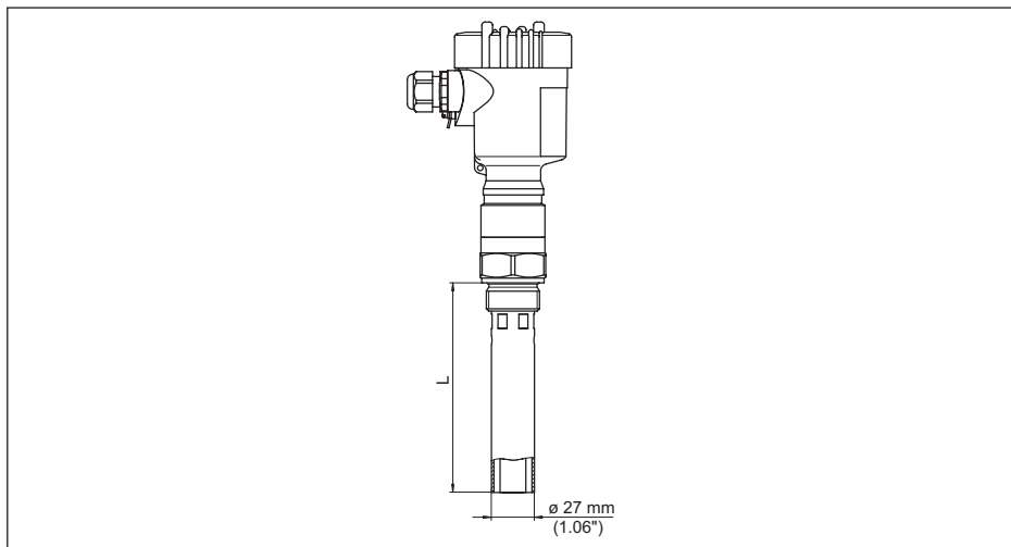
Abb. 37: VEGACAL 62, Hüllrohr z. B. bei kleiner Dielektrizitätszahl oder zur Linearisierung
