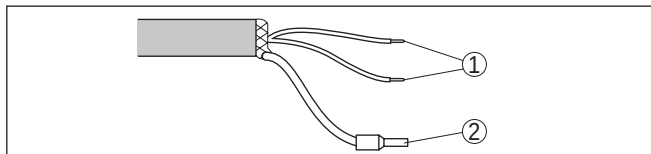
Abb. 20: Aderbelegung Anschlusskabel
