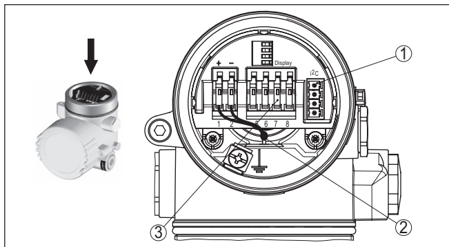
Abb. 13: Elektronikraum - Zweikammergehäuse
