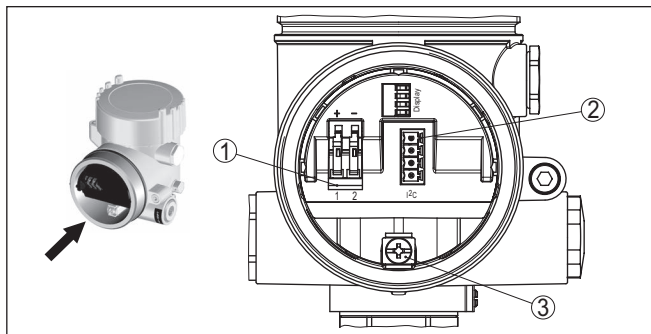
Abb. 14: Anschlussraum - Zweikammergehäuse
