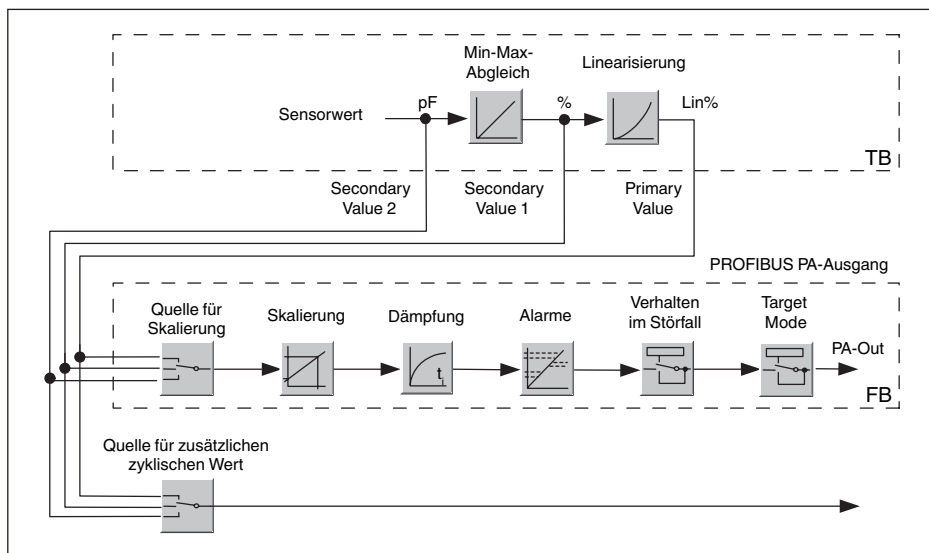
Abb. 29: VEGACAL 62: Blockschaltbild mit AI (PA-OUT)-Wert und zusätzlichem zyklischen Wert
