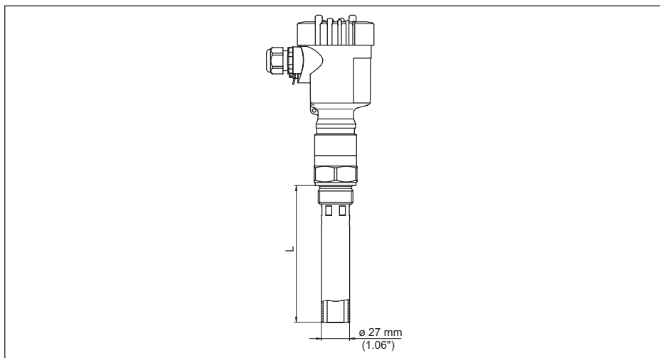
Abb. 36: VEGACAL 63, Hüllrohr z. B. bei kleiner Dielektrizitätszahl oder zur Linearisierung
