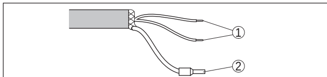
Abb. 20: Aderbelegung Anschlusskabel
