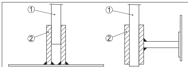
Abb. 6: Messsonde fixieren
