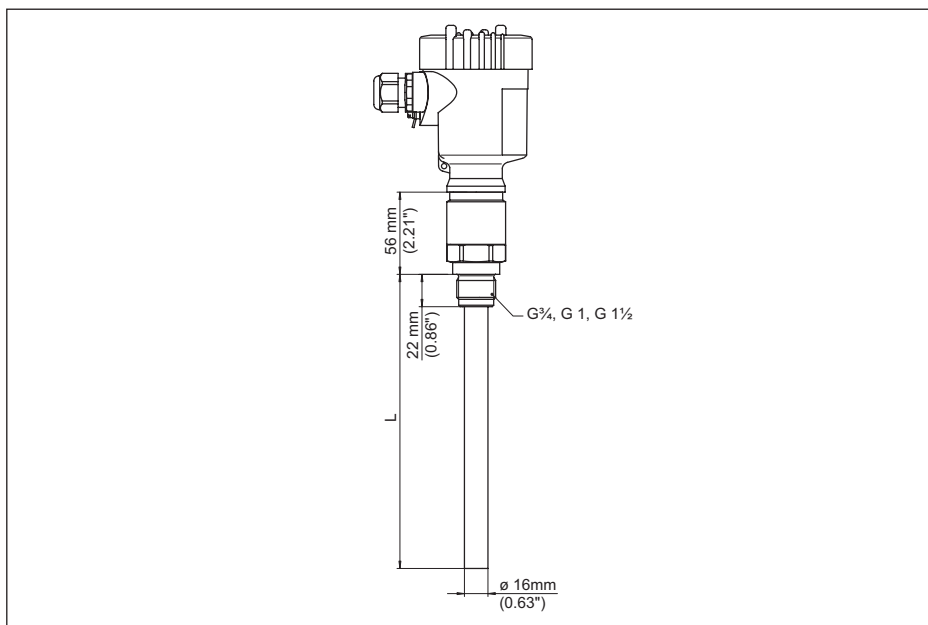
Figura 34: VEGACAL 63, esecuzione filettata G1 (ISO 228 T1)
