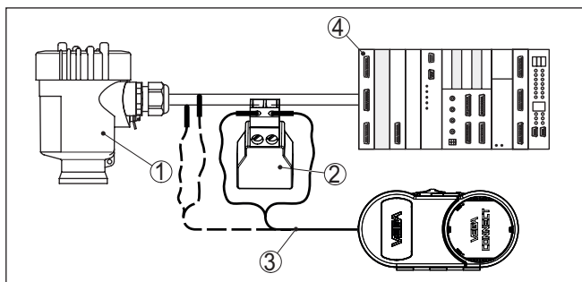
Fig. 25: Aansluiting van de PC via HART op de signaalkabel
