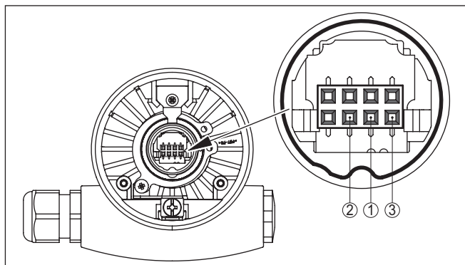
Fig. 29: Weerstand binnen de sensor controleren
