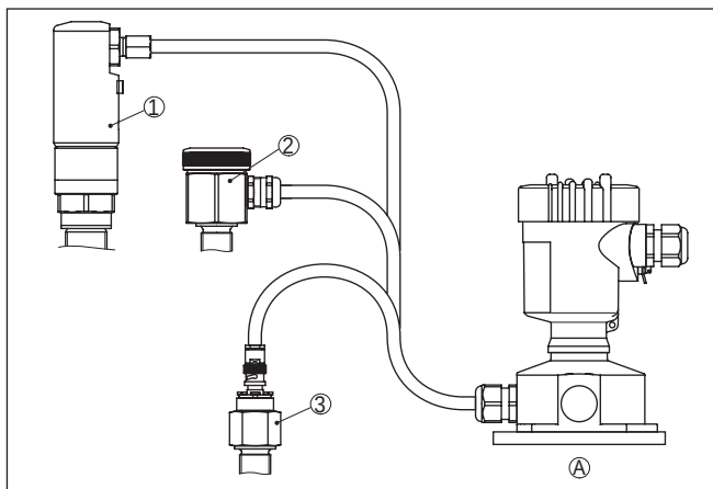
Fig. 4: Externe behuizing
