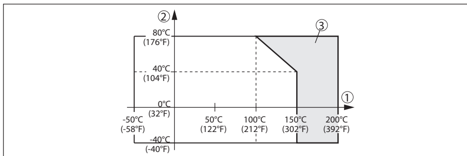
Fig. 30: Omgevingstemperatuur - procestemperatuur
