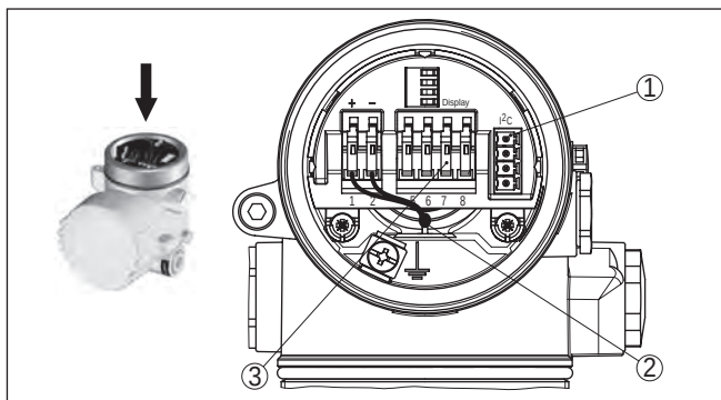
Abb. 13: Elektronikraum - Zweikammergehäuse
