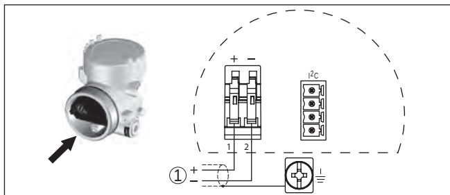
Abb. 15: Anschlussplan - Zweikammergehäuse
