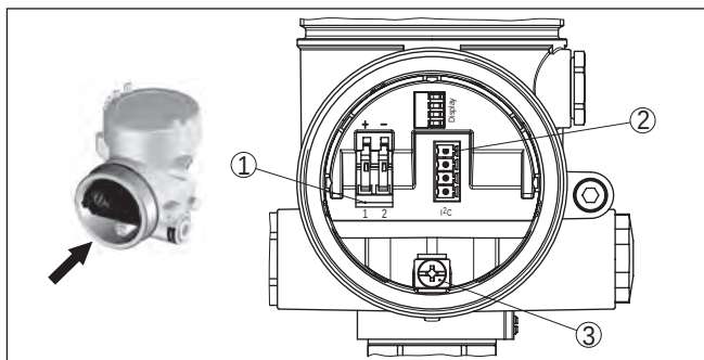
Abb. 14: Anschlussraum - Zweikammergehäuse
