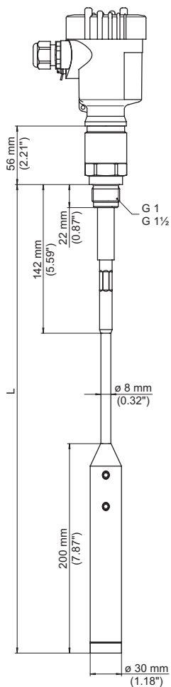
Figura 36: VEGACAL 65, esecuzione a fune con \varnothing 8 mm (0.315 in), esecuzione filettata G1 (ISO 228 T1)
