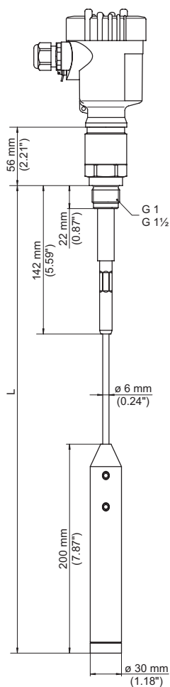
Figura 35: VEGACAL 65, esecuzione a fune con \varnothing 6 mm (0.236 in), esecuzione filettata G1 (ISO 228 T1)
