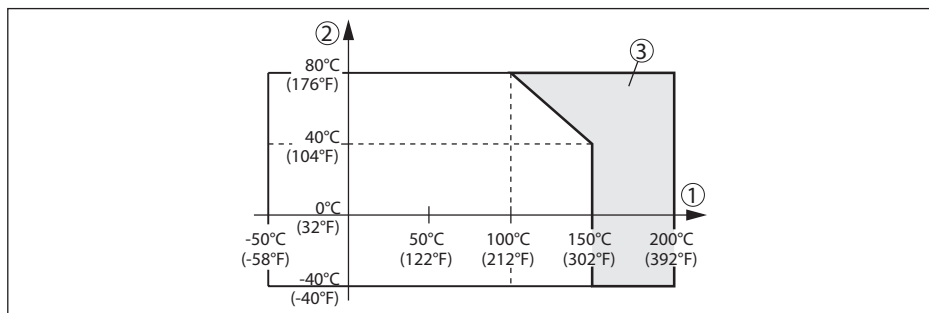
Figura 31: Temperatura ambiente - Temperatura di processo
