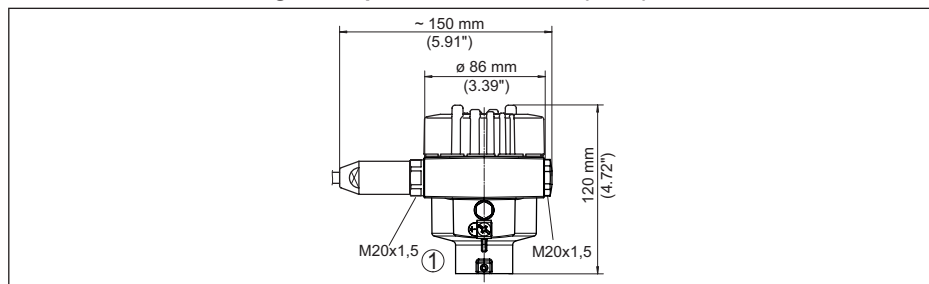
Figura 34: Differenti custodie con grado di protezione IP66/IP68 (1 bar), (con tastierino di taratura con display incorporato l'altezza della custodia aumenta di 18 mm/0.71 in)
