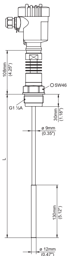
Figura 37: VEGACAL 65, Fune isolata in PTFE ( \varnothing 8 mm) con puntale a crimpare / -50 ... +200 °C
