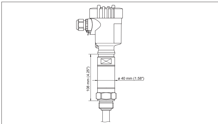
Figura 38: Pezzo intermedio di isolamento termico
