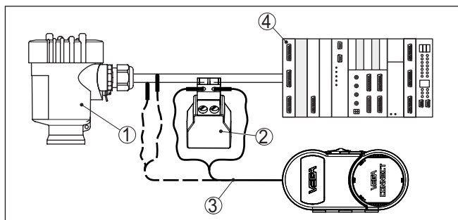
Figura 25: Collegamento del PC via HART alla linea del segnale
