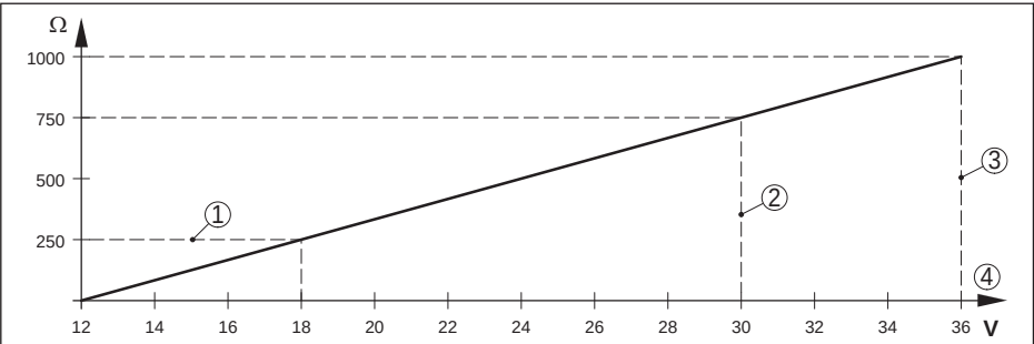
Abb. 31: Spannungsdiagramm
