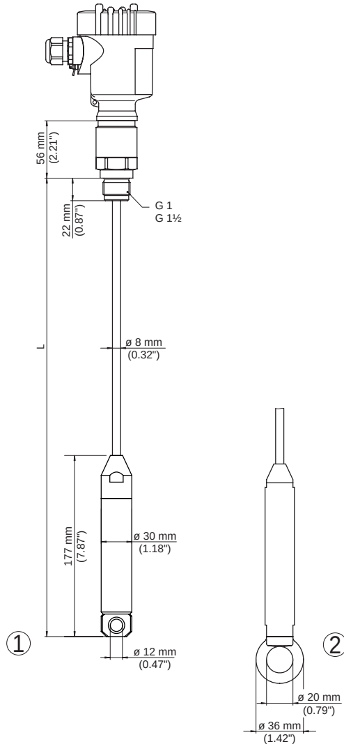
Abb. 34: VEGACAL 66, Gewindeausführung G1 (ISO 228 T1)
