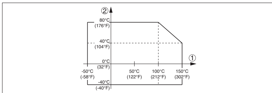
Abb. 30: Umgebungstemperatur - Prozesstemperatur
