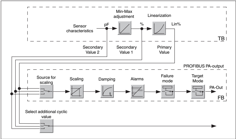
插图. 29: VEGACAL 66 : 带有 AI (PA-OUT) 值和额外的周期值的方块图
