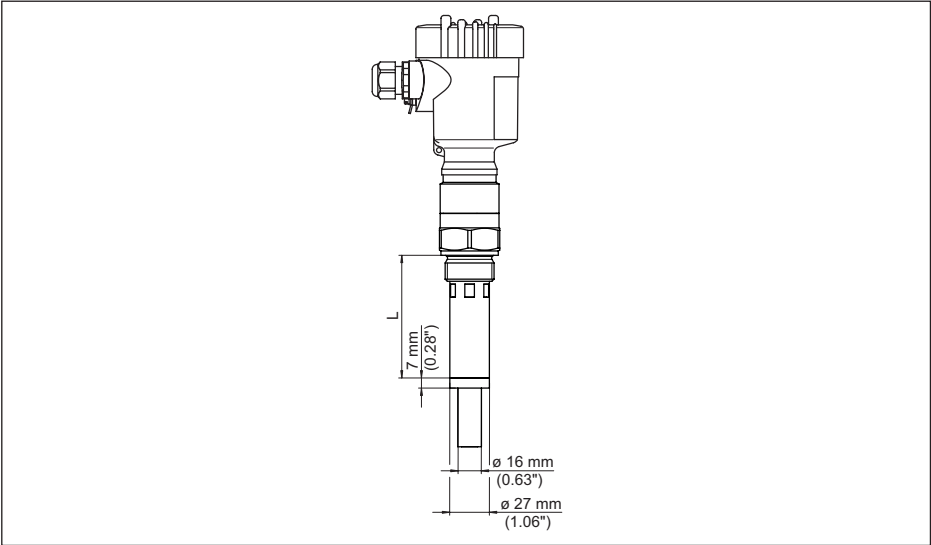
插图. 35: VEGACAL 66, 屏蔽管, 如用于防止冷凝水大量积聚
