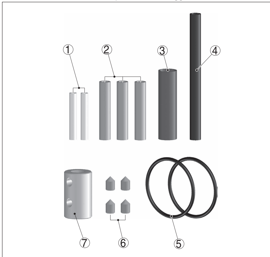
Figura 1: Kit per accorciamento della fune del VEGAVIB 62
