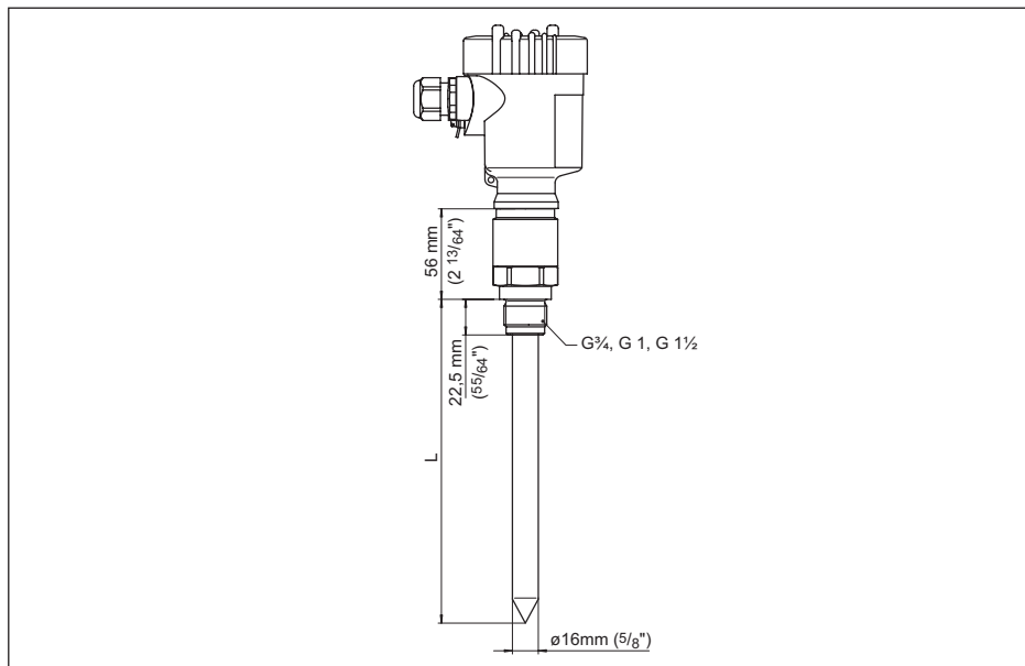
Abb. 19: VEGACAL 64, Gewindeausführung G1 (ISO 228 T1)
