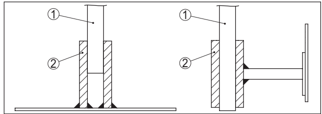
Abb. 6: Messsonde fixieren
