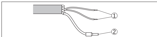
Abb. 12: Aderbelegung Anschlusskabel
