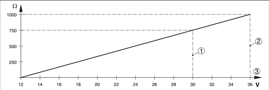
Abb. 16: Spannungsdiagramm
