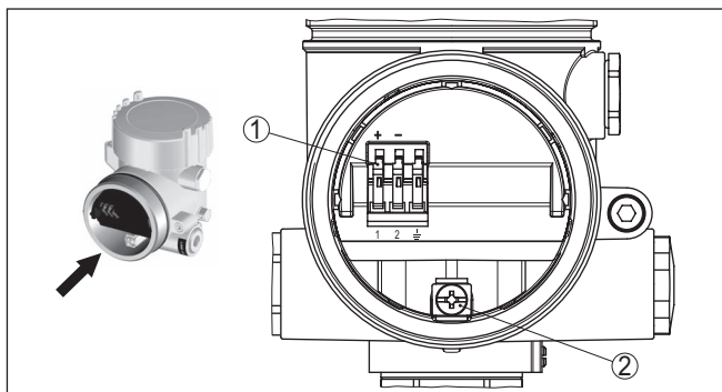
Abb. 17: Anschlussraum Ex-d-ia-Zweikammergehäuse
