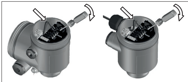
Abb. 7: Anschlusschritte 6 und 7
