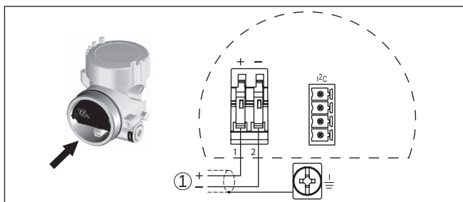
Abb. 14: Anschlussplan - Zweikammergehäuse
