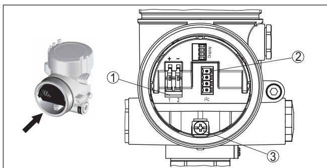
Abb. 13: Anschlussraum - Zweikammergehäuse
