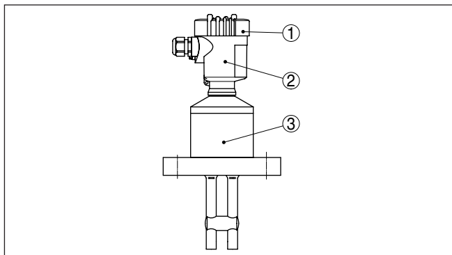
Abb. 1: VEGACAL 69 - Zweistabmesssonde mit Kunststoffgehäuse
