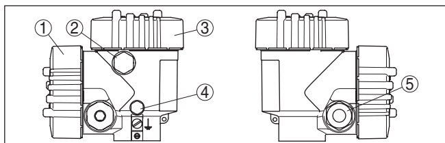
Abb. 11: Zweikammergehäuse
