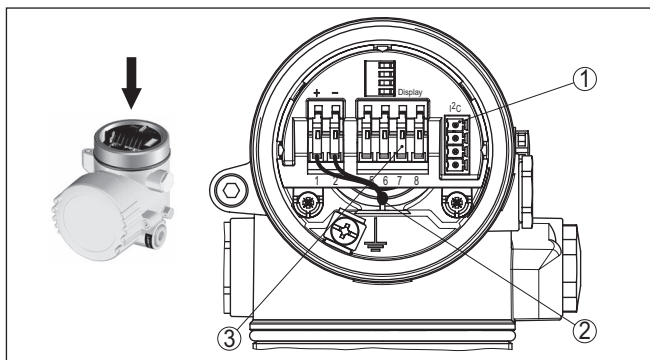
Abb. 12: Elektronikraum - Zweikammergehäuse
