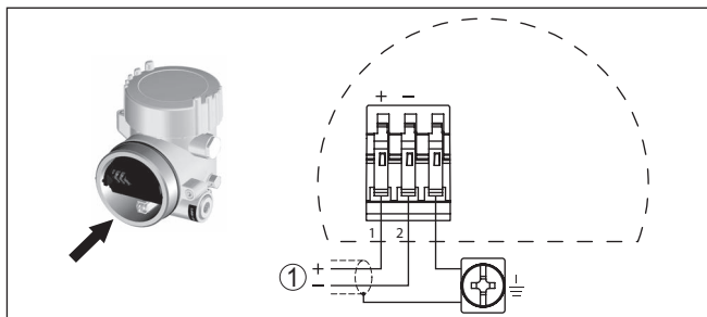
Abb. 18: Anschlussplan Ex-d-ia-Zweikammergehäuse
