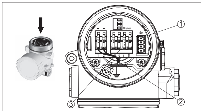
Abb. 16: Elektronikraum - Zweikammergehäuse
