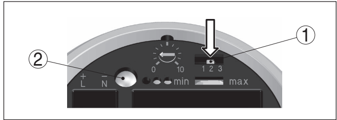
Fig. 16: Compensatieknop
