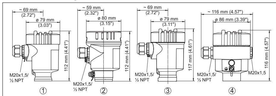
Fig. 18: Uitvoeringen behuizing
