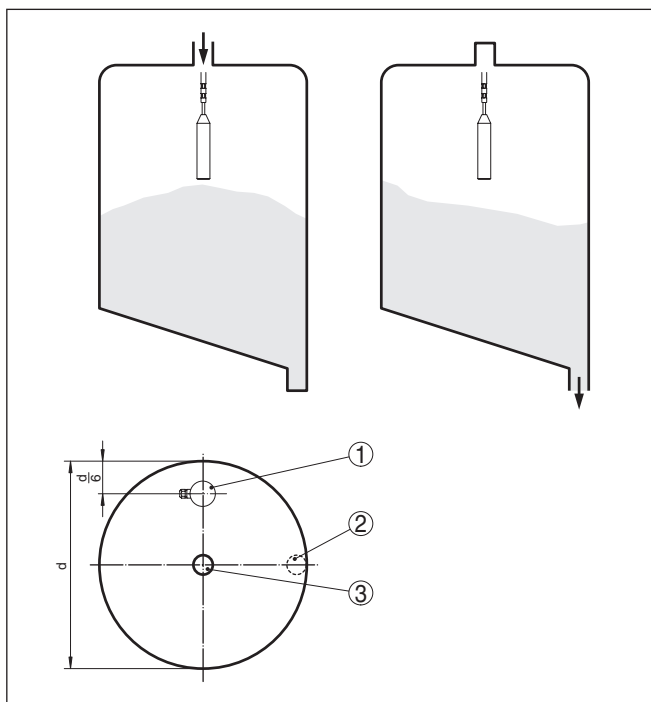
Fig. 7: Vullen in het midden, afvoer aan de zijkant
