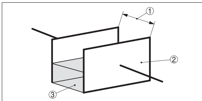
Fig. 3: Werkingsprincipe - plaatcondensator
