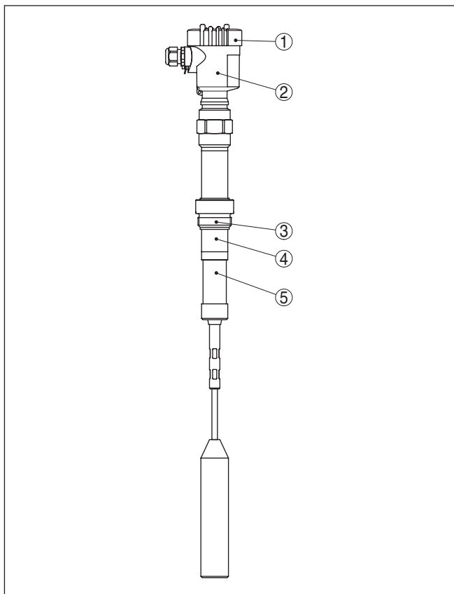
Fig. 1: VEGACAP 67 met kunststof behuizing
