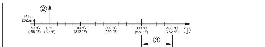
Fig. 17: Procestemperatuur - procesdruk
