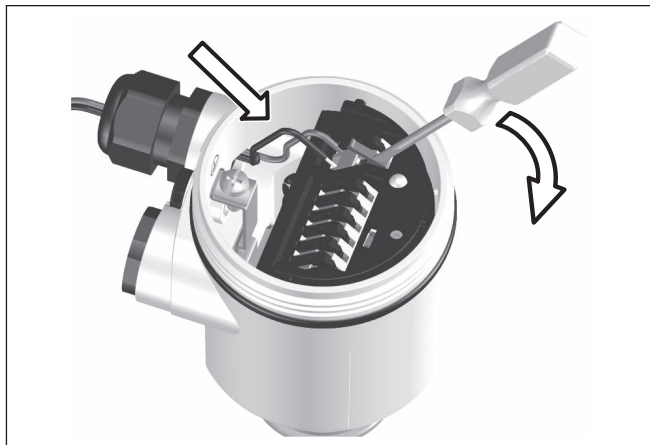
Fig. 8: Pasos de conexión 5 y 6
