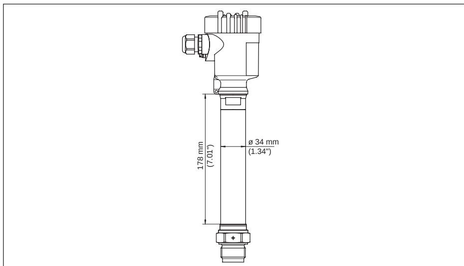
Fig. 33: Temperatuurtussenstuk
