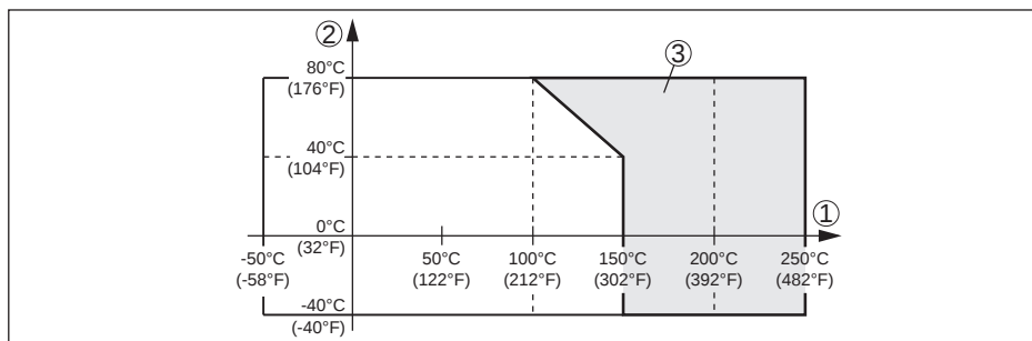
Fig. 30: Omgevingstemperatuur - procestemperatuur
