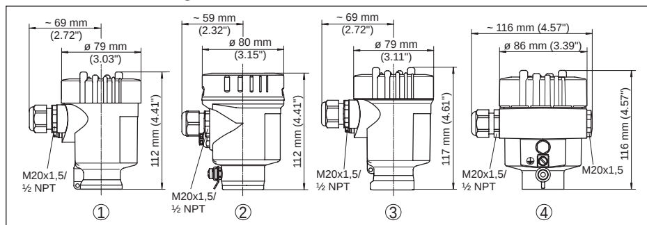
Fig. 31: Uitvoeringen behuizing
