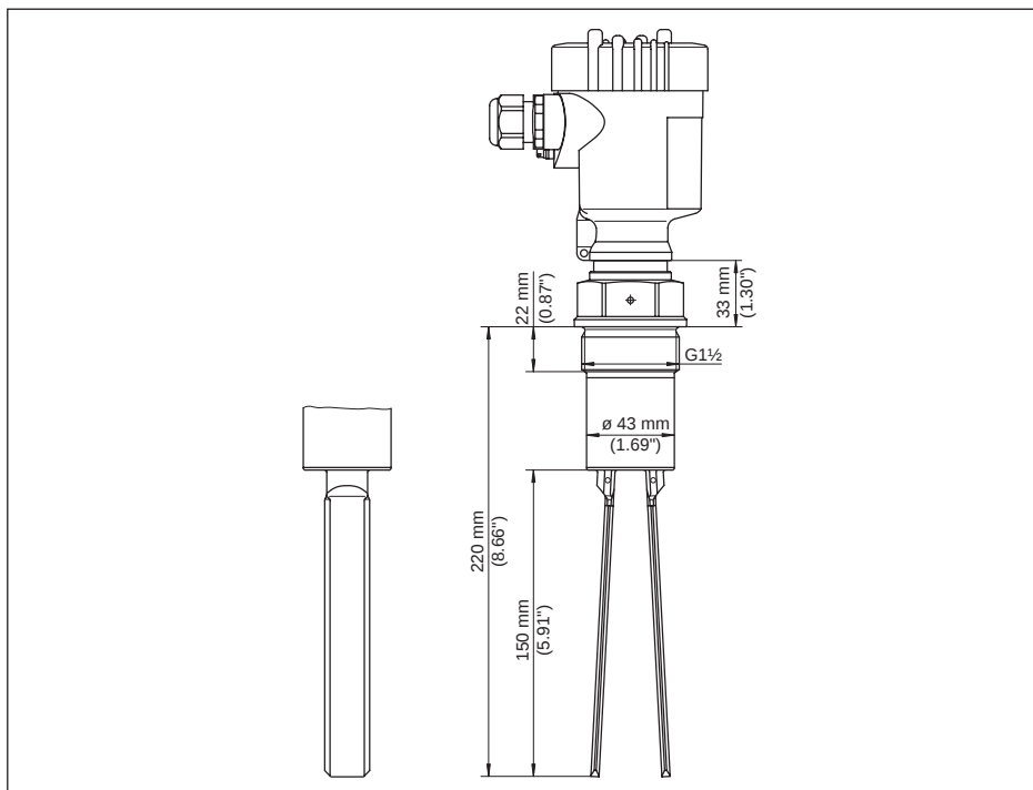
Fig. 32: VEGAWAVE 61, schroefdraaduitvoering G1½ (DIN ISO 228/1)
