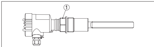
Fig. 6: Montaje horizontal - marca
