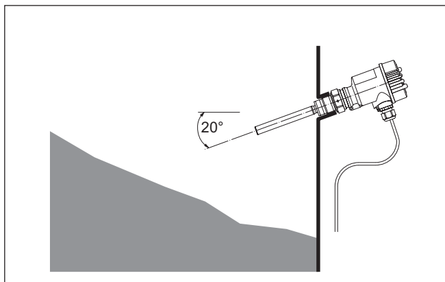
Fig. 4: Montaje horizontal
