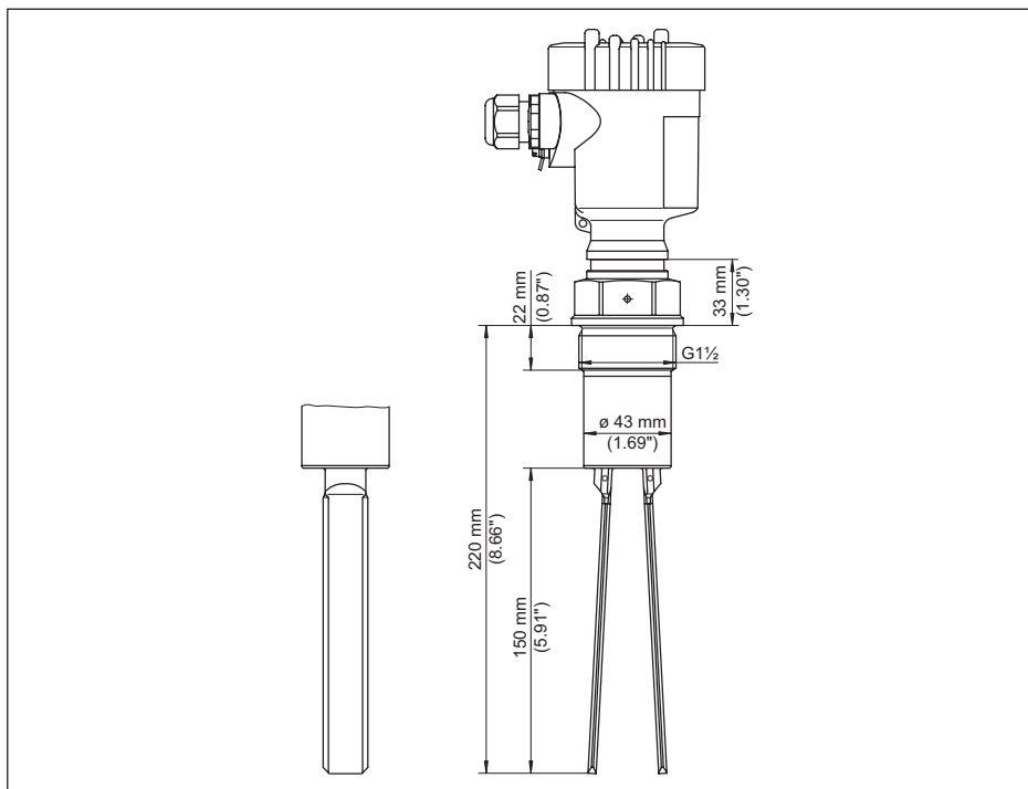
Fig. 16: VEGAWAVE 61, versión roscada G1½ (DIN ISO 228/1)
