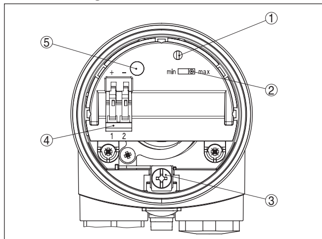
Fig. 12: Elektronica- en aansluitruimte - tweedraadsuitgang
