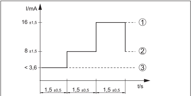
Fig. 13: Verlooptiagram van de functietest (bedrijfsmodus "max")
