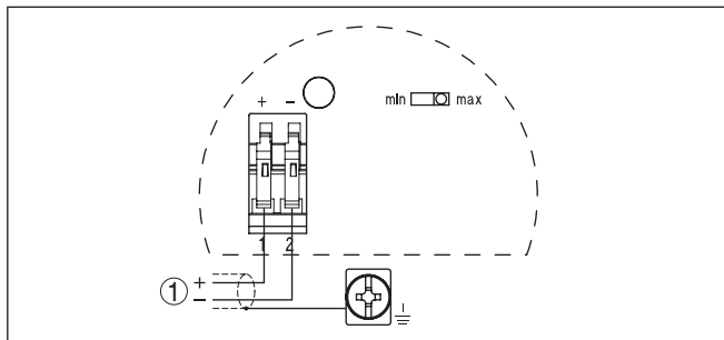
Fig. 10: Aansluitschema
