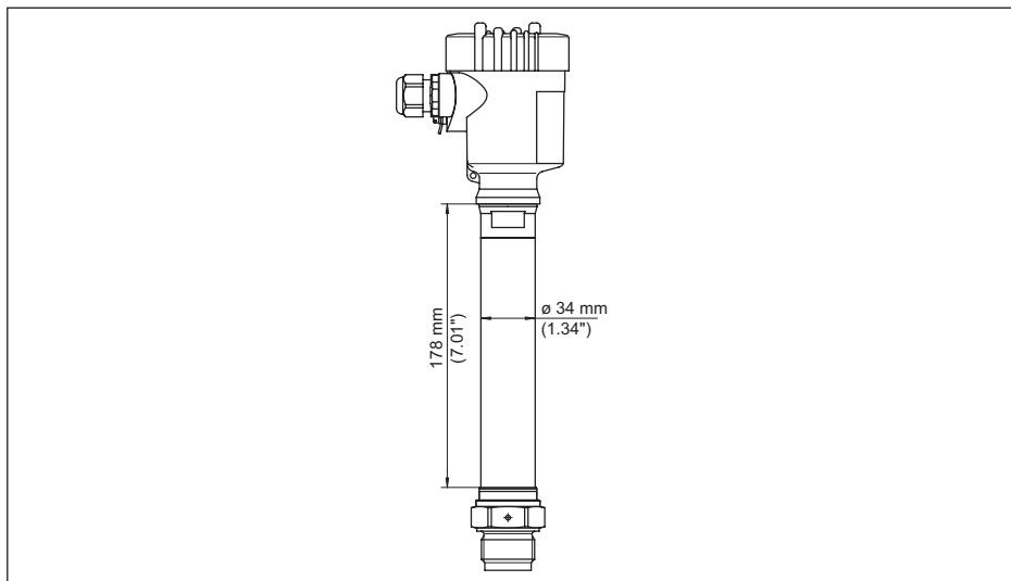
Fig. 20: Temperatuurtussenstuk
