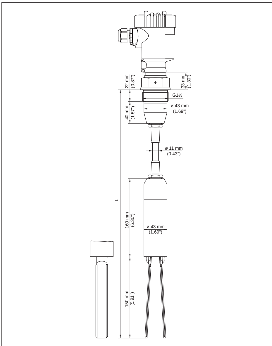
Abb. 30: VEGAWAVE 62 mit PUR-Tragkabel, Gewindeausführung G1½ (DIN ISO 228/1)
