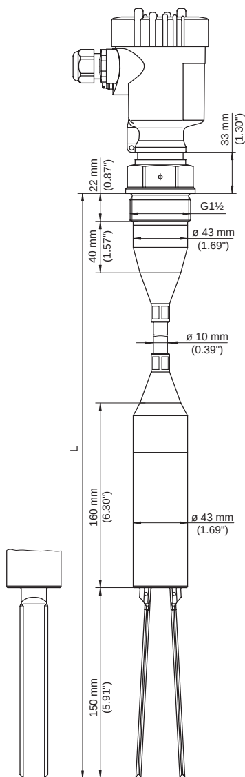
Abb. 31: VEGAWAVE 62 mit FEP-Tragkabel, Gewindeausführung G1½ (DIN ISO 228/1)
