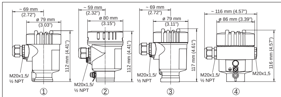
Abb. 29: Gehäuseausführungen
