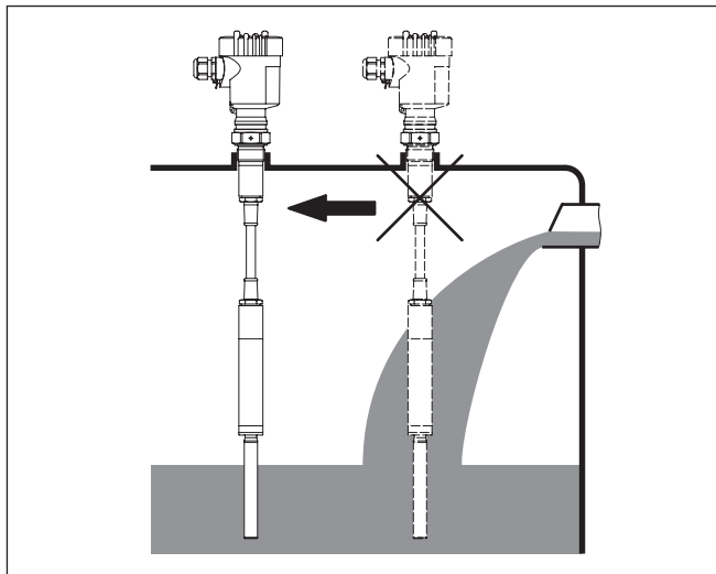
Abb. 5: Einstömendes Medium
