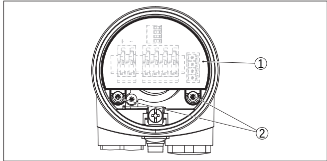
Abb. 28: Halteschrauben lösen
