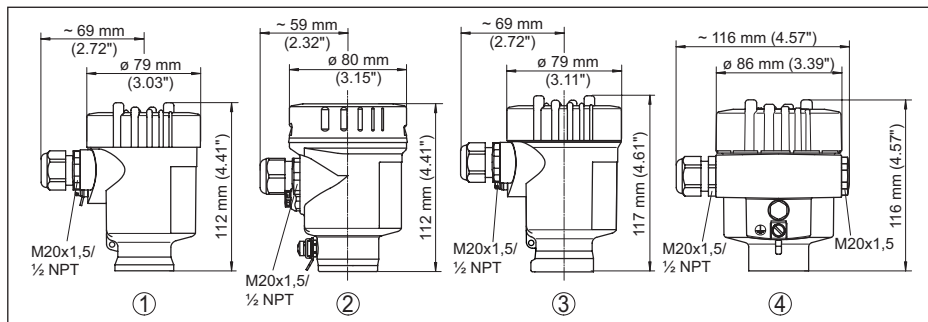
Fig. 13: Uitvoeringen behuizing
