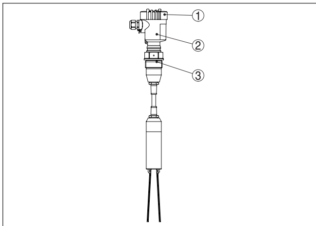
Fig. 1: VEGAWAVE 62 met kunststof behuizing
