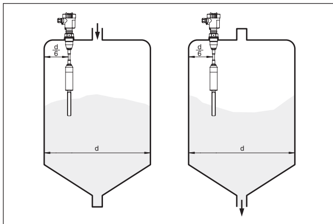
Fig. 3: Vullen en afvoeren in het midden
