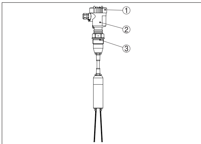
Fig. 1: VEGAWAVE 62 avec boîtier en plastique
