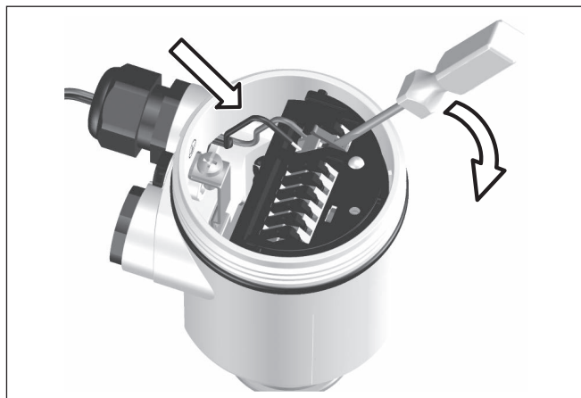
Fig. 8: Étapes de raccordement 5 et 6
