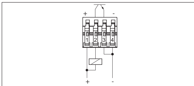
Fig. 11: Comportement NPN
