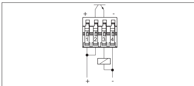
Fig. 12: Comportement PNP
