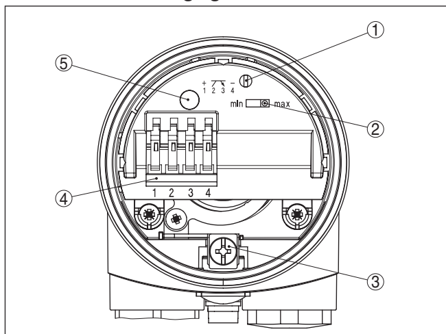
Fig. 14: Compartiment électronique et de raccordement - sortie transistor
