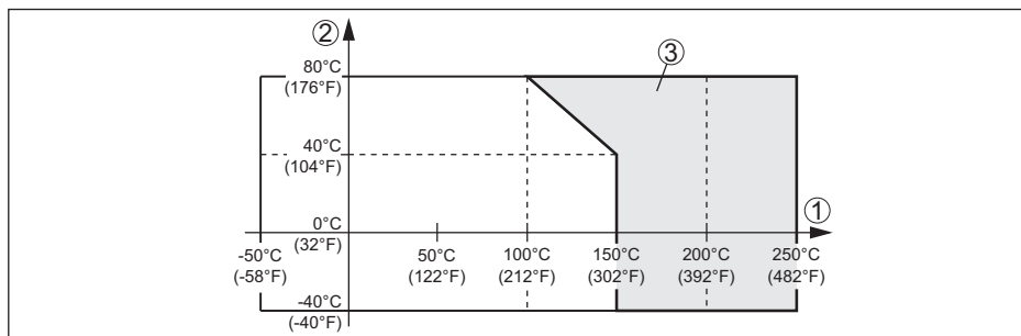
Fig. 14: Omgevingstemperatuur - procestemperatuur
