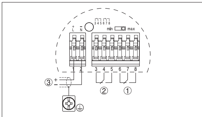
Fig. 10: Aansluitschema
