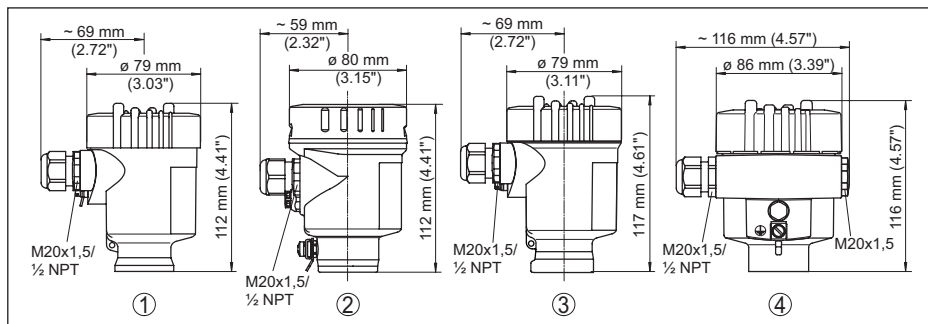
Fig. 15: Uitvoeringen behuizing
