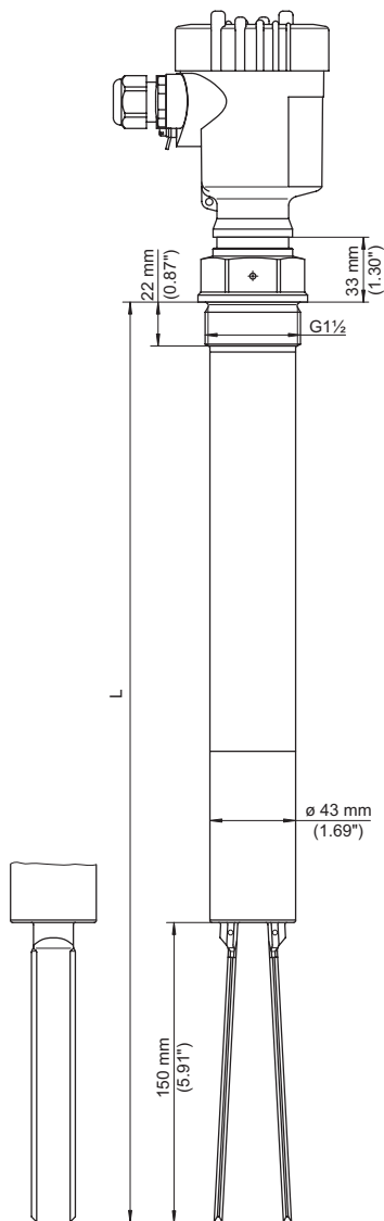
Fig. 16: VEGAWAVE 63, schroefdraaduitvoering G1½ (DIN ISO 228/1)
