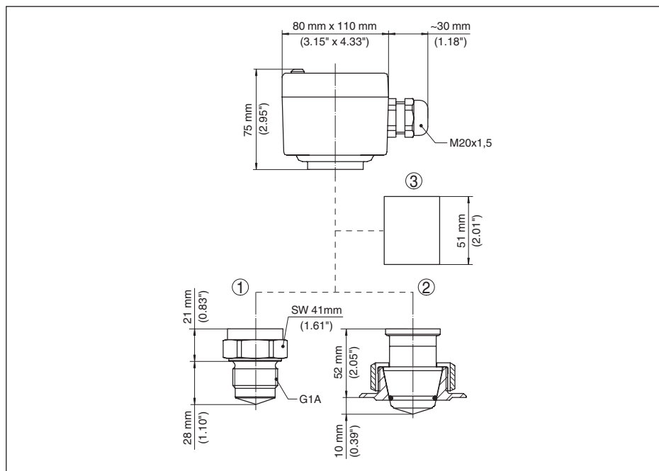
Fig. 19: VEGAKON 61
