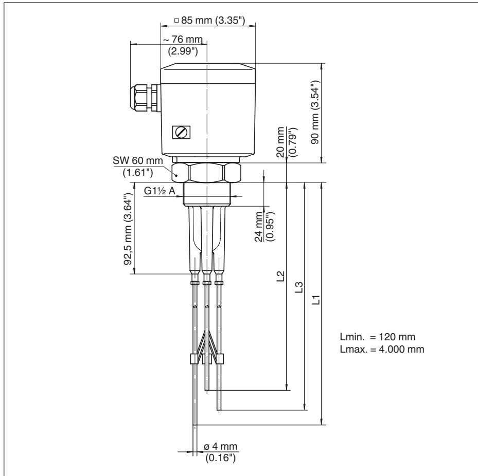
Fig. 8: VEGAKON 66 met drie elektroden
