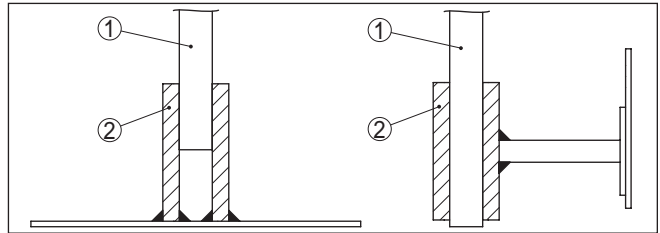
Fig. 4: Meetsonde fixeren
