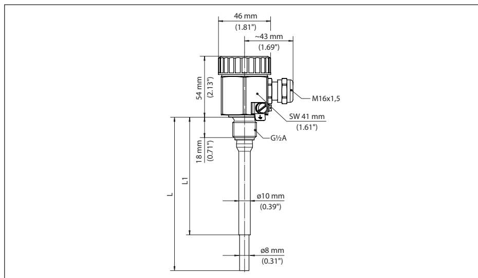
Fig. 8: Sonde de mesure résistive à tige EL 1
