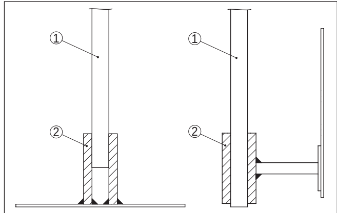
Abb. 3: Messsonde fixieren
