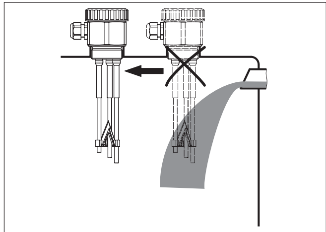
Abb. 4: Einströmendes Medium
