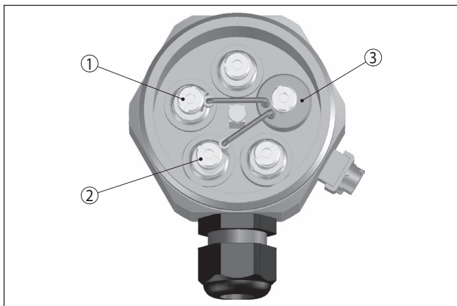
Abb. 6: Montage der Zusatzelektronik zur Leitungsbruchüberwachung
