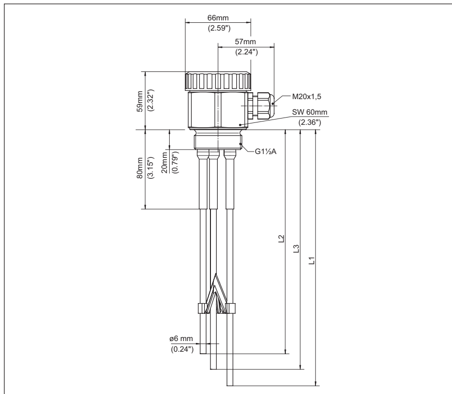
Figura 7: Sonda conduttiva a più barre EL 3
