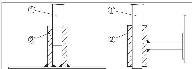
Fig. 3: Meetsonde fixeren
