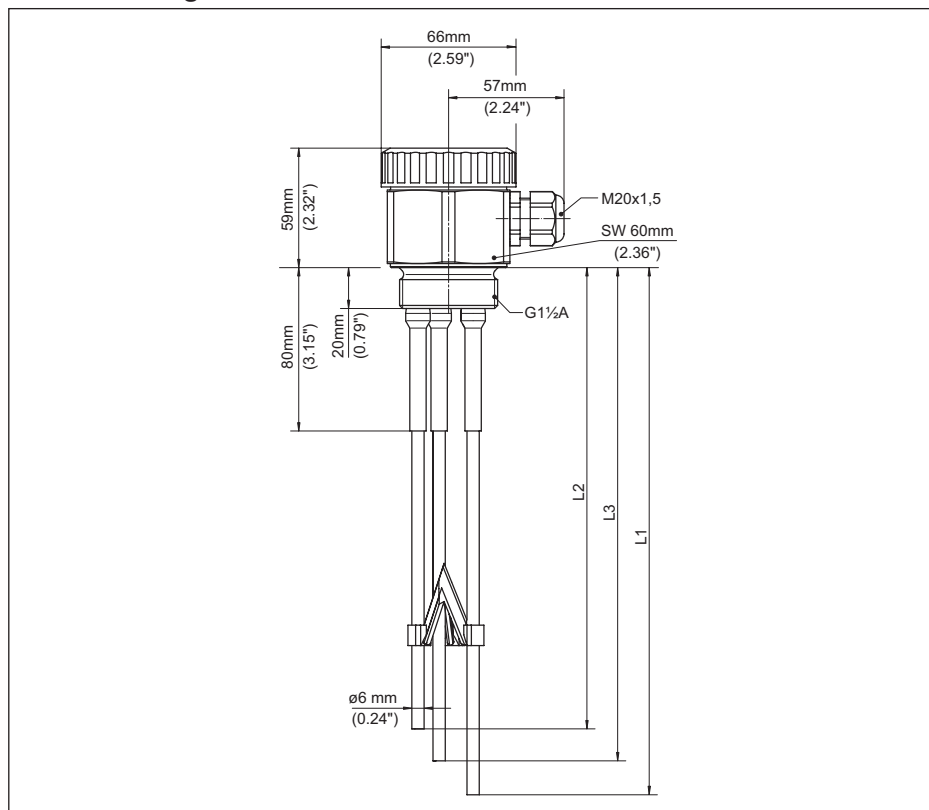
Fig. 7: Conductieve meerstaafs-meetsonde EL 3
