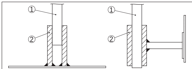
插图. 3: 将测量探头固定好
