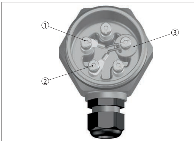
插图. 6: 请为电线断裂监控安装附加电子部件
