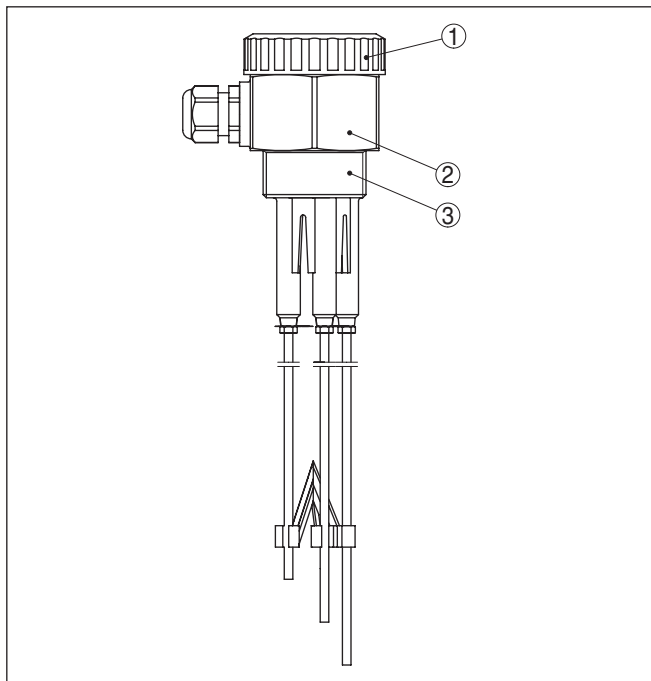
插图 1: 导电性多棒式测量探头 EL 4
