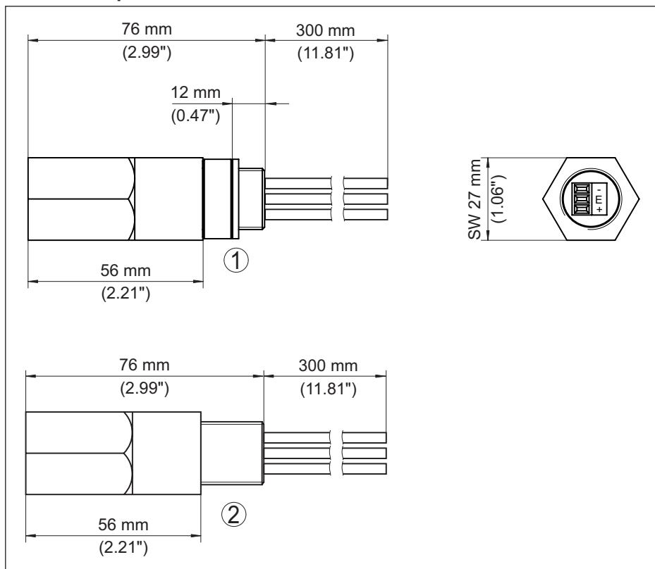
Рис. 4: Размеры B63-48, B63-32
