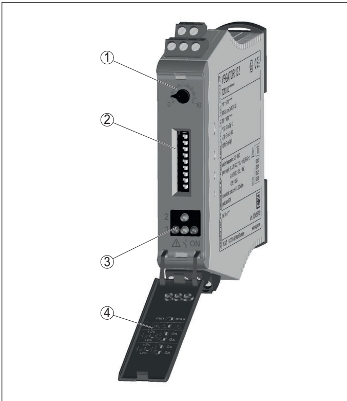
Abb. 18: Anzeige- und Bedienelemente am Beispiel des VEGATOR 132
