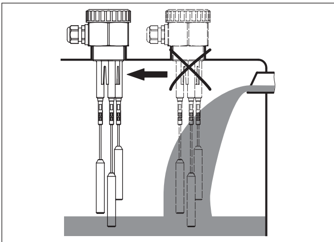
Abb. 5: Einströmendes Medium
