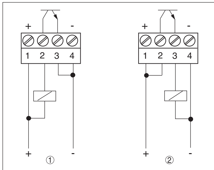
Abb. 12: VEGAKON 66 - Elektronik mit Transistorausgang
