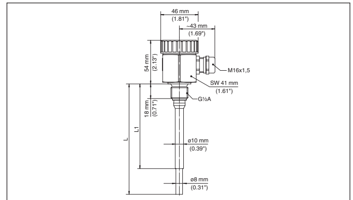
Abb. 21: Konductive Stabmesssonde EL 1
