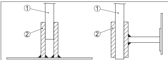
Abb. 4: Messsonde fixieren
