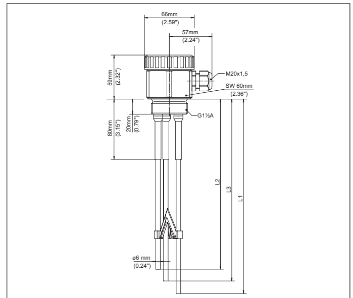
Abb. 22: Konductive Mehrstabmesssonde EL 3
