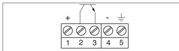
Abb. 9: VEGAKON 61 - Transistorausgang
