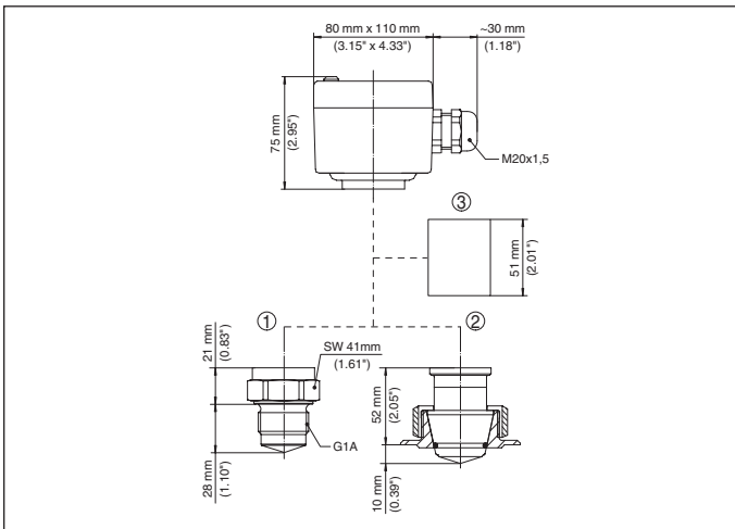
Abb. 19: VEGAKON 61
