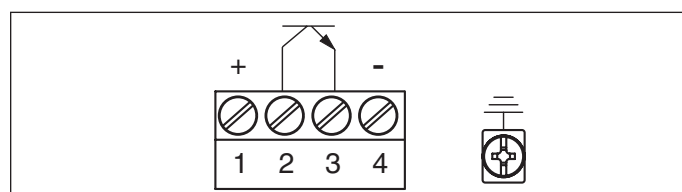
Abb. 10: VEGAKON 66 - Transistorausgang
