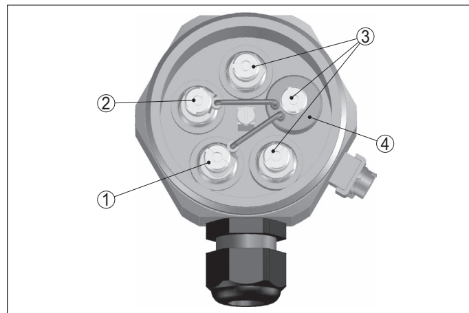
Abb. 13: Zusatzelektronik zur Leitungsbruchüberwachung in Verbindung mit VEGATOR 131, 132
