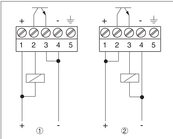
Fig. 18: VEGAKON 61 - elektronica met transistoruitgang
