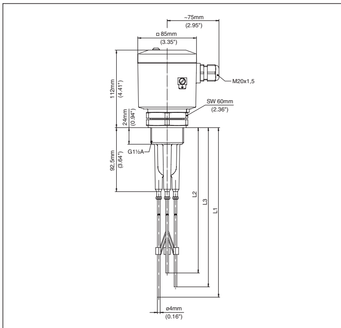
Fig. 27: VEGAKON 66 met drie elektroden
