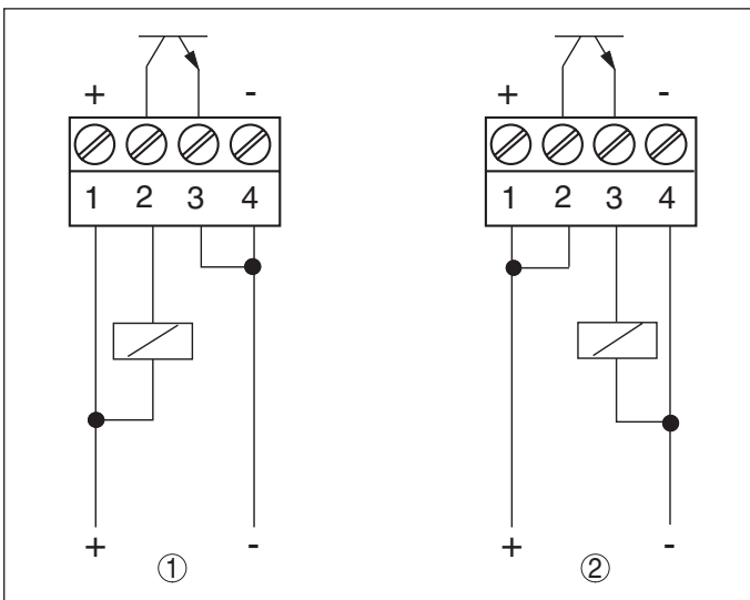
Fig. 19: VEGAKON 66 - elektronica met transistoruitgang
