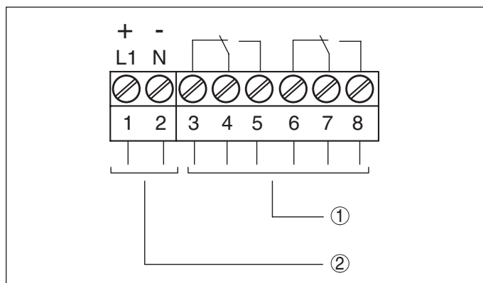
Fig. 15: VEGAKON 66 - elektronica met relaisuitgang
