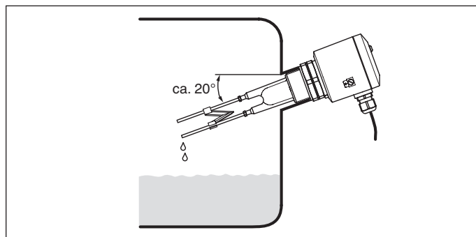
Fig. 13: Horizontale montage
