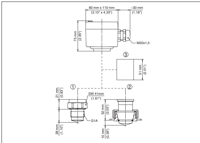
Fig. 26: VEGAKON 61
