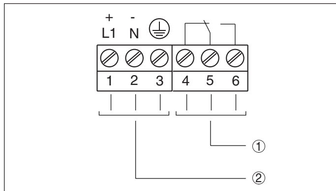
Fig. 14: VEGAKON 61 - elektronica met relaisuitgang
