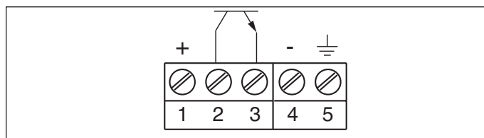
Fig. 16: VEGAKON 61 - transistoruitgang
