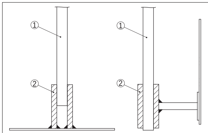
Fig. 11: Meetsonde fixeren
