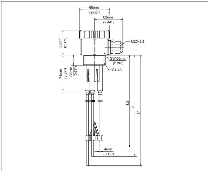
Fig. 30: Conductieve meerstaafs-meetsonde EL 4
