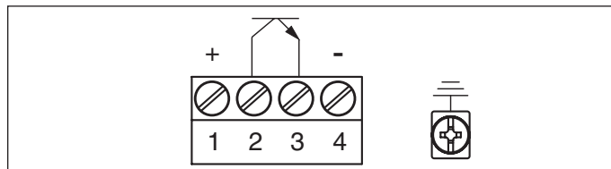
Fig. 17: VEGAKON 66 - transistoruitgang
