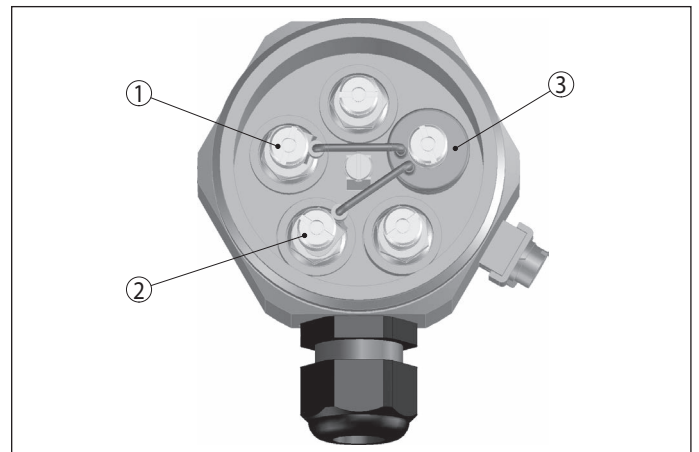
Fig. 21: Montage van de extra elektronica voor kabelbreukbewaking
