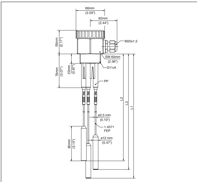
Fig. 31: Conductieve meerkabelmeetsonde EL 6
