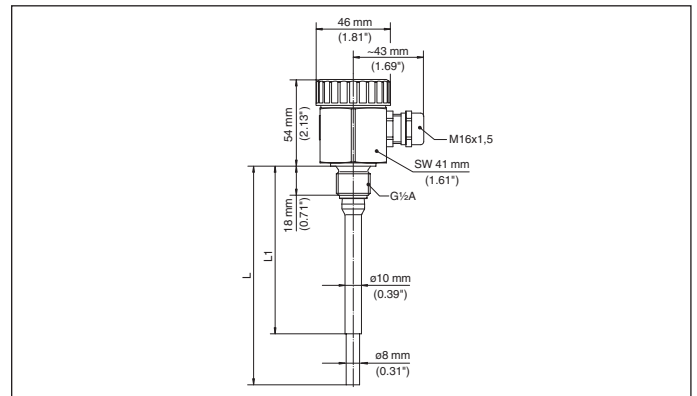
Fig. 28: Conductieve staafmeetsonde EL 1
