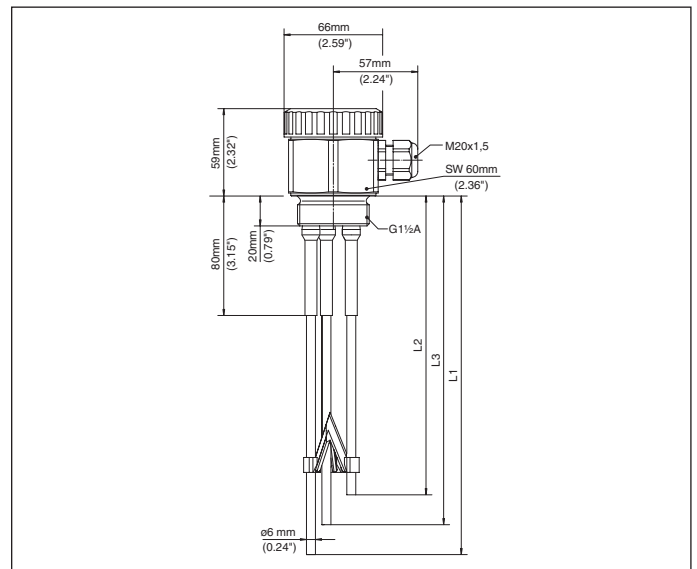
Fig. 29: Conductieve meerstaafs-meetsonde EL 3
